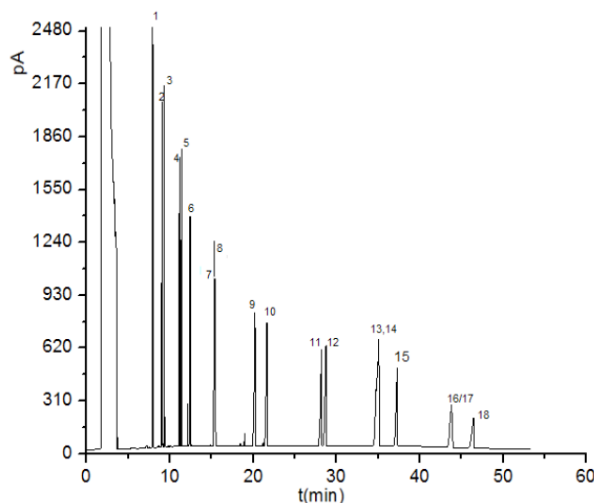
Gráfico 1. Cromatograma del patrón estándar de los 18 HAP (Restek EPA method 8310 PAH Mix
