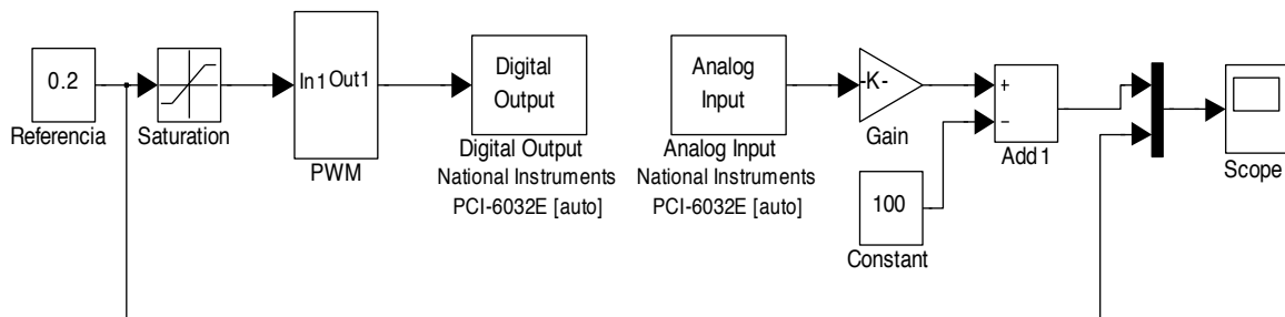
FIG. 3. Diagrama de bloques en lazo abierto para realizar la identificación de la planta
