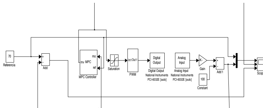
FIG. 12. Diagrama de bloques para el control experimental de temperatura MPC.
