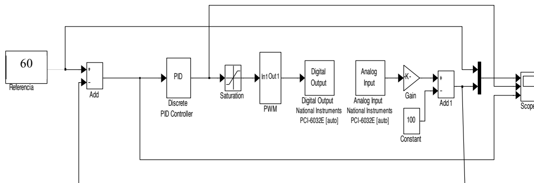
FIG. 10. Diagrama de bloques para el control experimental de temperatura PID
