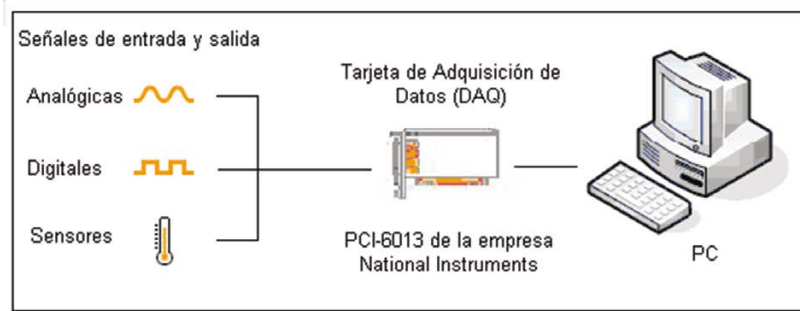
FIG. 2. Sistema de adquisición de datos
