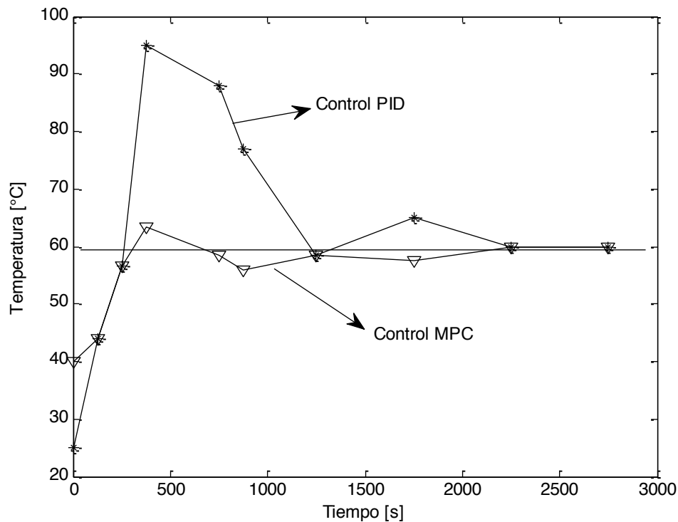
FIG. 14. Respuestas de los sistemas de control PID y MPC
