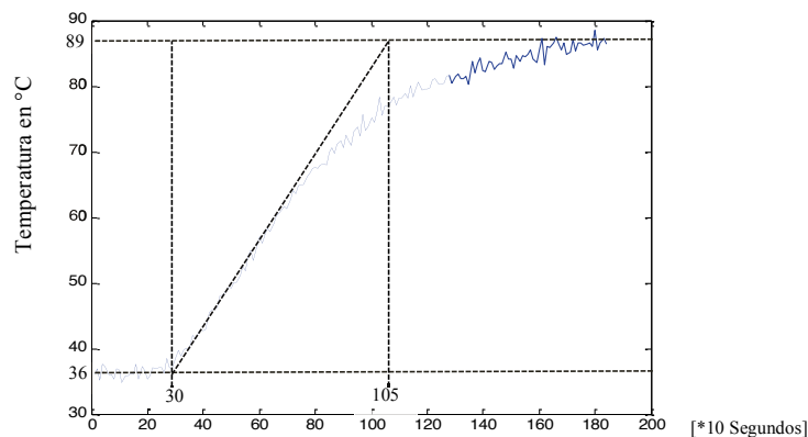
FIG. 4. Respuesta de la planta en lazo abierto
