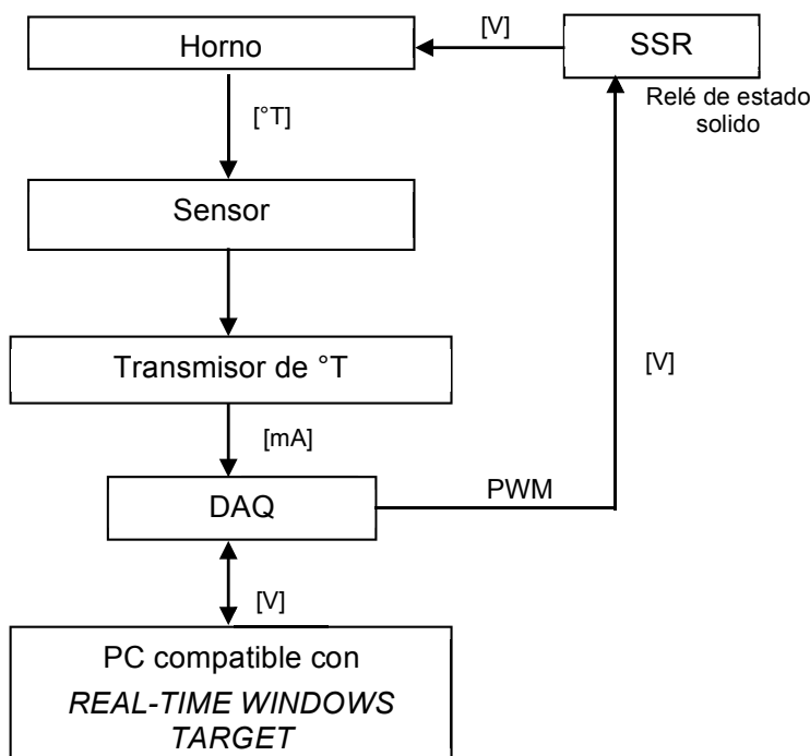
FIG. 1. Diagrama de bloque sistema de control de temperatura
