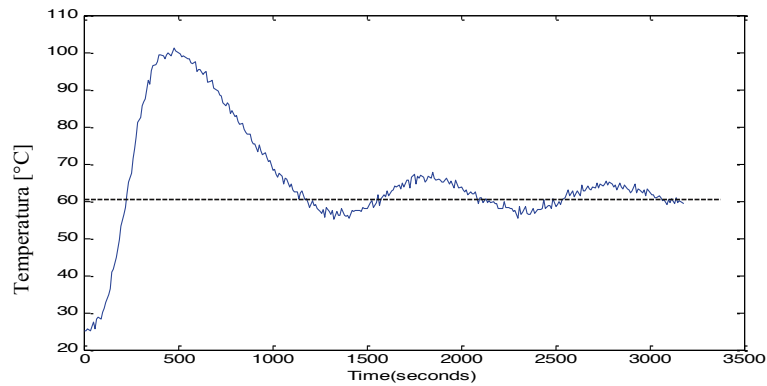
FIG. 11. Respuesta del sistema de control experimental PID de temperatura en lazo cerrado
