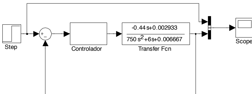
FIG. 8. Diagrama de bloques para el control de temperatura
