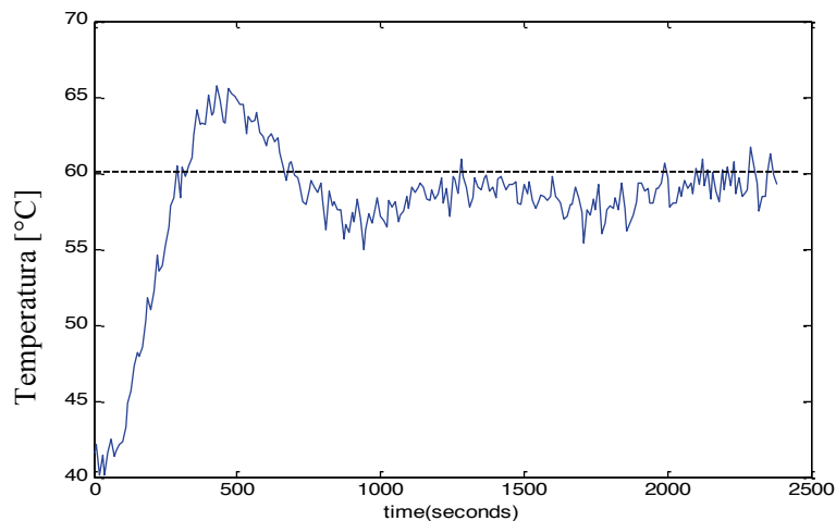
FIG. 13. Respuesta del sistema de control experimental MPC de temperatura en lazo cerrado
