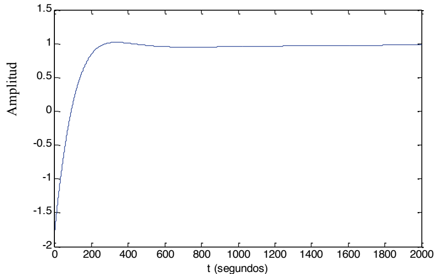
FIG. 9. Respuesta del sistema de simulación del control de temperatura PID.
