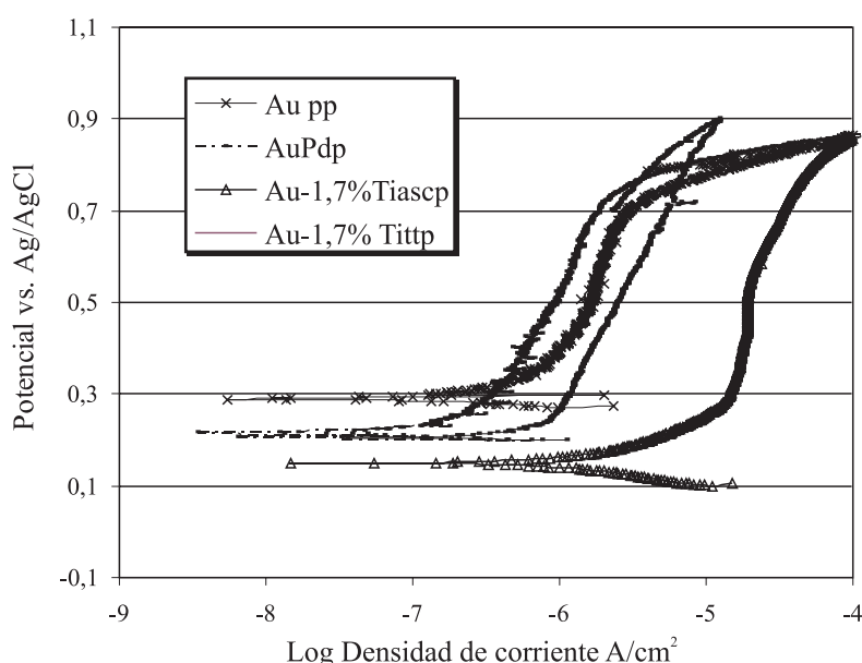
Figura 5 Curvas de segunda polarización para las muestras de oro puro pasivada (Au p), la aleación Au-Pd-Ga-In pasivada (AuPd), Au-1,7% Ti “as cast” pasivada (Au -1,7% Ti ascp) y Au-1,7% con 4 h de envejecimiento pasivada (Au- 1,7% Ti ttp). Todas las polarizaciones se realizaron en solución de Ringer desaireada a 37 °C
