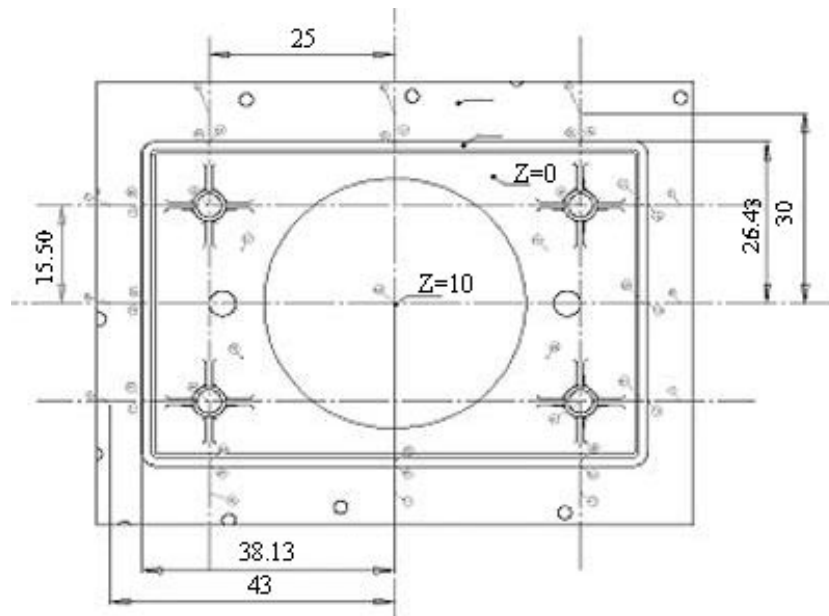
Figura 4 Cotas definidas para la pieza base
