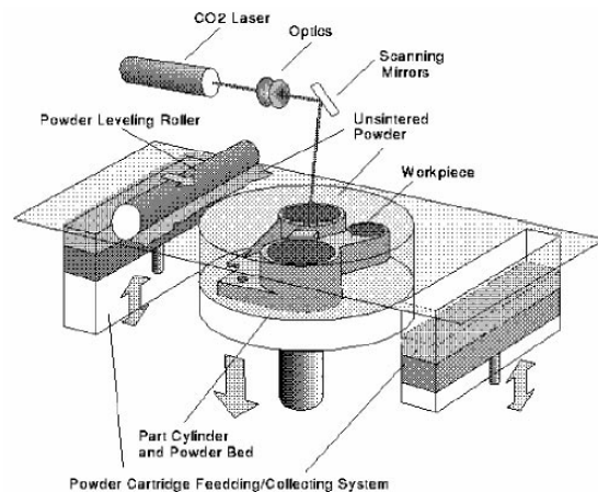
Figura 8 Esquema del funcionamiento de la máquina SLS
