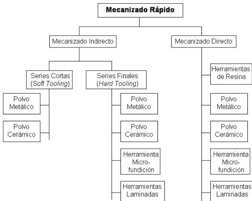
Figura 1 Clasificación de los métodos de rapid tooling [5]
