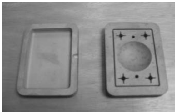
Figura 9 Insertos SLS-pieza tapa y pieza base
