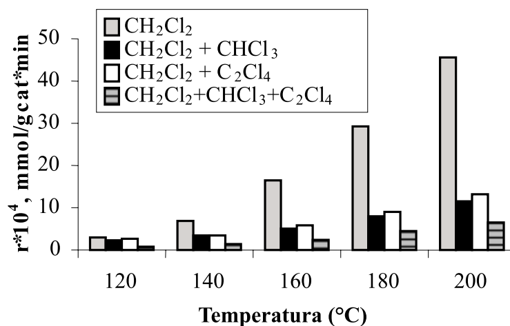
Figura 11 Comparación entre las mezclas, binarias y ternarias de diclorometano con trazas de cloroformo y tetracloroetileno. Catalizador: 0,6% Pd/ \gamma -Al 2 O 3 . 25 mg de catalizador, v_o = 120 mL/min
