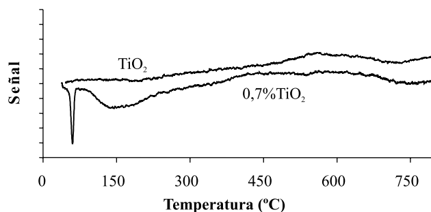
Figura 7 Perfiles TPR de los catalizadores frescos: \text{TiO}_2 y 0,7% \text{Pd/TiO}_2 sol-gel
