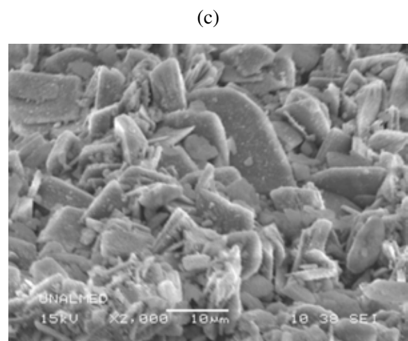
Figura 5 a, b, c. Micrografías del producto comercial (SEM)
