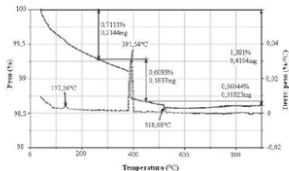
Figura 7 Análisis térmico diferencial y termogravimétrico para la hidroxiapatita UdeA a 850 °C
