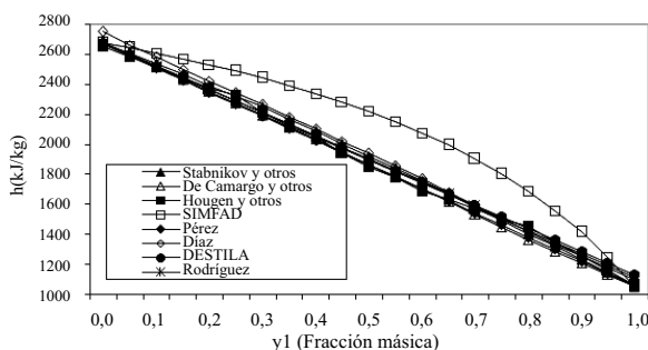
Figura 12 Entalpía de la mezcla como vapor saturado
