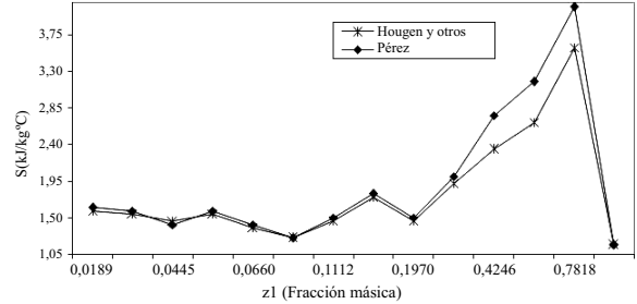
Figura 19 Entropía de la mezcla como mezcla húmeda
