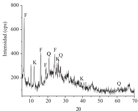
Figura 3 Difractograma de Rayos X del FCC (F: faujasita, Q: cuarzo, K: caolinita)
