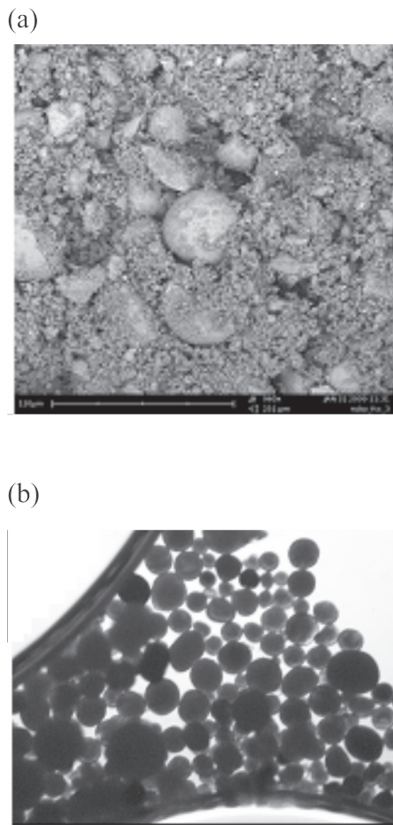
Figura 2 Imágenes del FCC: a) Tomada por MEB, b) Tomada por microscopía óptica
