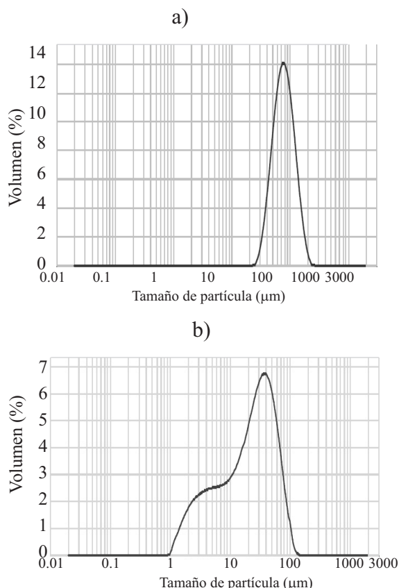
Figura 1 Ensayo de granulometría láser del FCC a) antes y b) después del proceso de molienda
