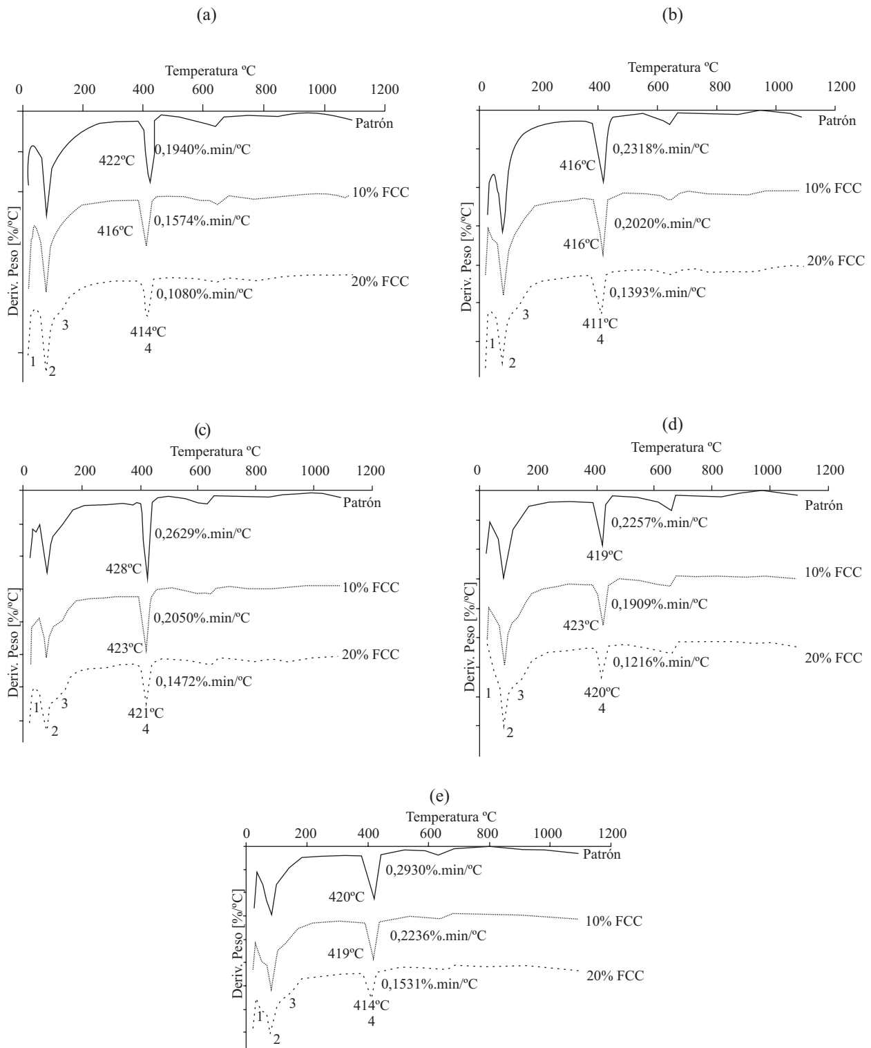
Figura 5 Curvas DTG a diferentes edades de curado. a) 1 día, b) 3 días, c) 8 días, d) 15 días y e) 28 días
