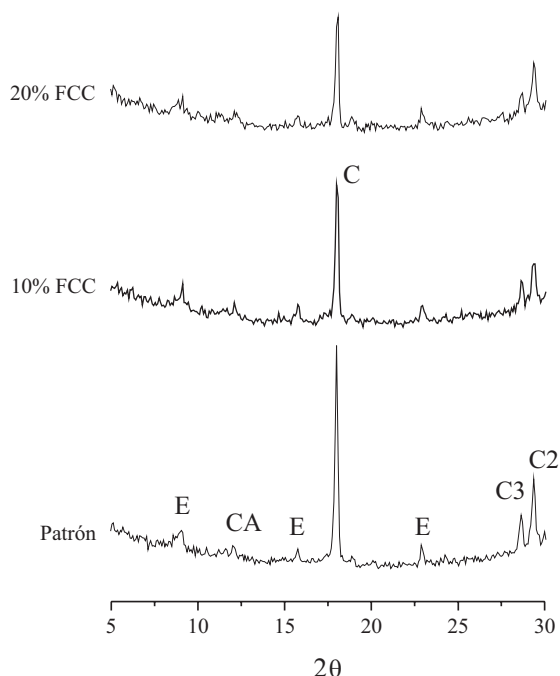
Figura 6 DRX de las pastas de OPC adicionadas con FCC: E: Ettringita, CA: CAH_{10} , C: Ca(OH)_2 , C3: Silicato tricálcico ( SC_3 ), C2: Silicato bicálcico ( SC_2 )
