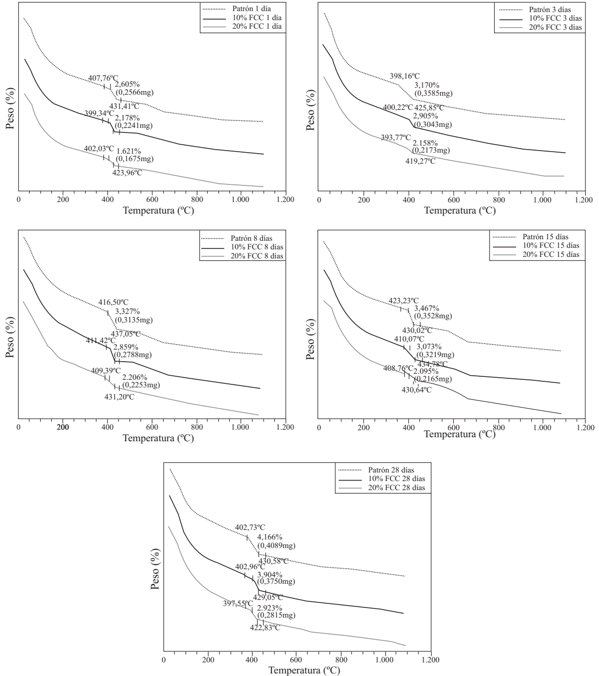
Figura 4 Curvas TG a diferentes edades de curado a 1, 3, 8, 15 y 28 días
