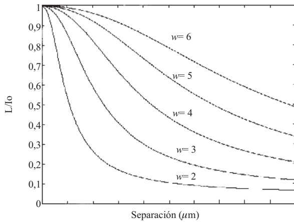
Figura 5 Intensidad reflejada sin interferencia para \lambda = 1,55\mu\text{m} (en orden decreciente w = 6, 5, 4, 3, 2\mu\text{m} )
