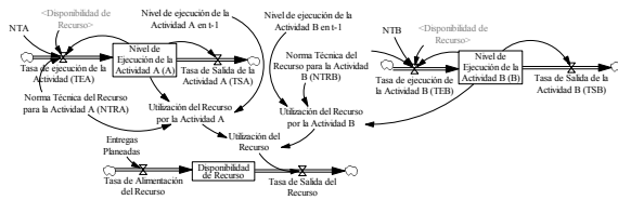
Figura 6 Representación forrester de recursos no renovables
