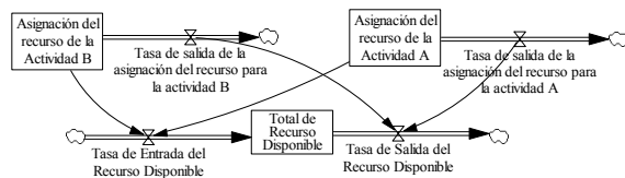
Figura 7 Representación forrester de los recursos renovables
