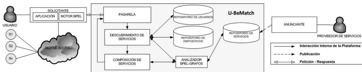
Solicitante: módulo compuesto por una aplicación móvil y un motor BPEL. La aplicación ofrece la interfaz gráfica para la interacción con el usuario, además de proveer las capacidades de comunicación para el envío y recepción de los
