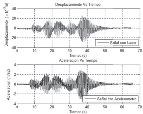
Figura 12 Prueba No.3: Registros en el tiempo
