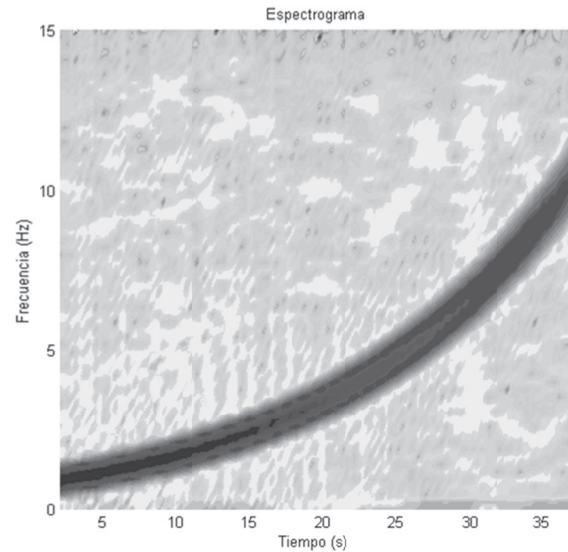
Figura 11 Prueba No.2: espectrograma para la señal del sistema láser
