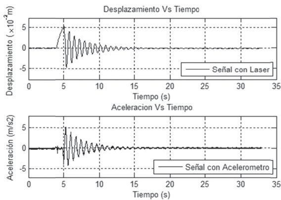
Figura 7 Prueba No.1: Registros en el tiempo
