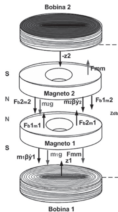
Figura 2 Diagrama de Fuerzas
