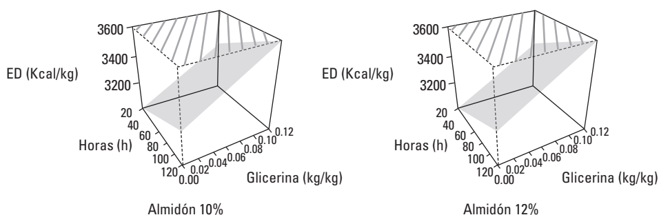
FIGURA 1. Relación entre la tasa de inclusión de glicerina cruda en la dieta (Glicerina), la duración del tránsito (Horas) y el valor de EDA corregida por el almidón de la dieta (ED) determinada por la TBMN.
