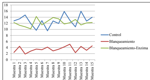
Figura 2. Comportamiento de los valores en Mpa de la resistencia de unión al corte por grupo
