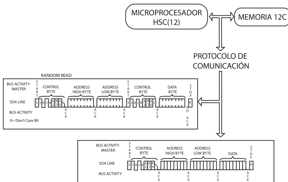
Figura 4. PROTOCOLO i2c [5]
