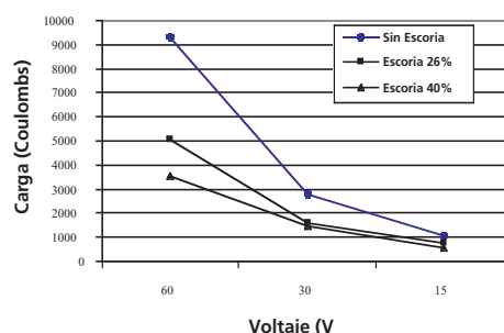
Figura 5. Carga total vs. voltaje utilizado para los diferentes porcentajes de adición. Relación agua cemento (a/c) de 0.84 y 50 días de edad.
