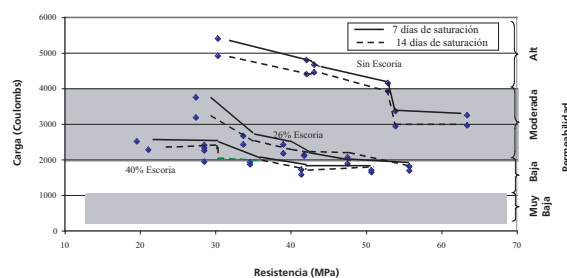
Figura 7. Carga total vs. resistencia a compresión a los 56 días para los dos tiempos de saturación.
