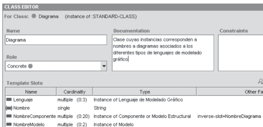
Figura 2. Propiedades asociadas a la clase Diagrama .
