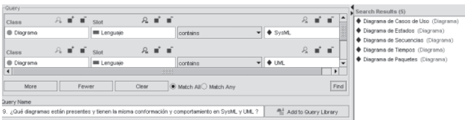
Figura 6. Resultado de la consulta 3.
