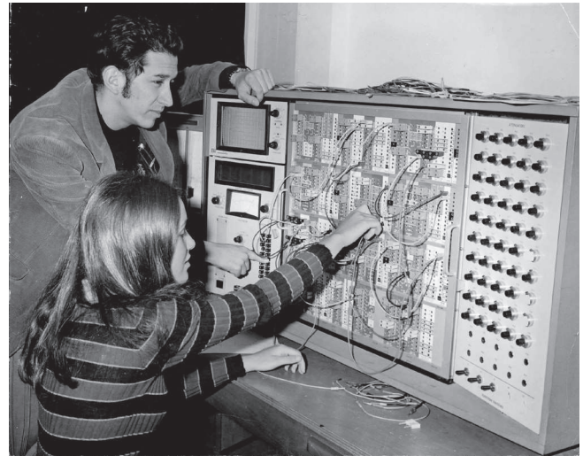
Foto 1 Computador análogo TR-48. Laboratorio de Ingeniería Electrónica. Edificio W.
