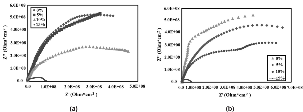
Figura 6. Diagramas de Nyquist para a) bronce, y b) latón, en un tiempo inicial ( t_0 )
