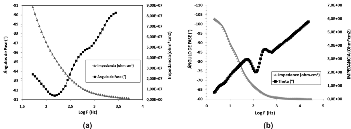
Figura 7. Espectros de Bode en gasolina pura a un tiempo de exposición inicial t_0 , para a) el latón y b) bronce
