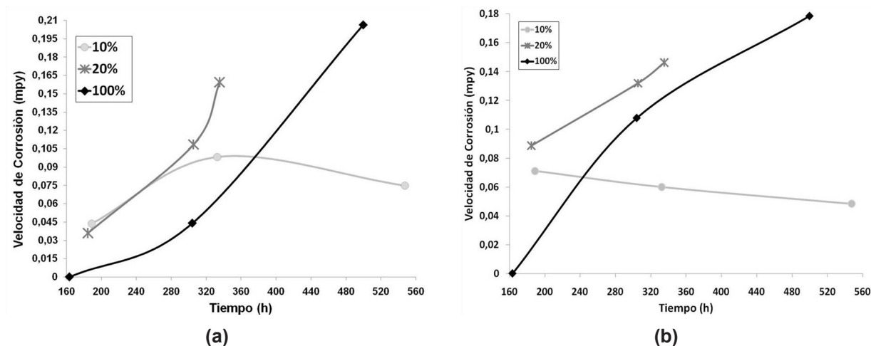
Figura 2. Curvas de la velocidad de corrosión vs tiempo a diferentes mezclas de bioetanol-gasolina para a) bronce, y b) latón
