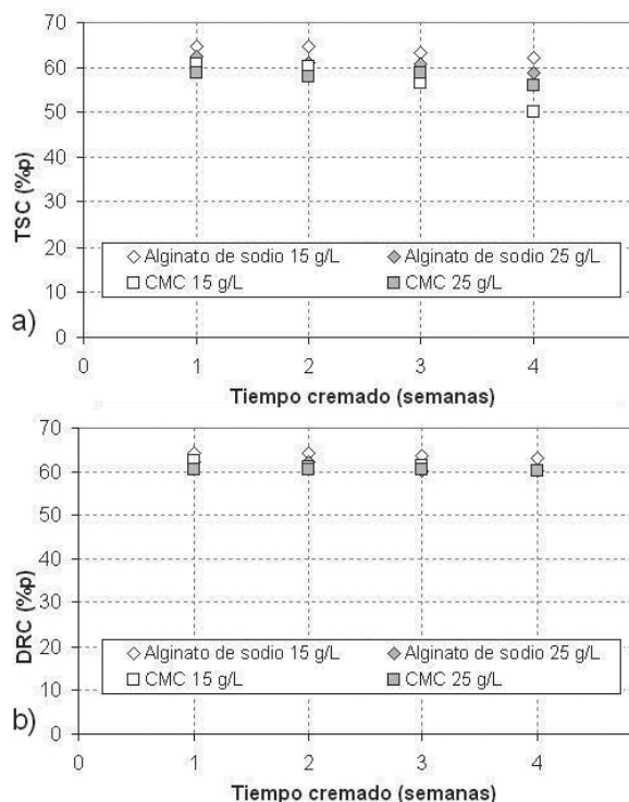
Figura 2. Figura 2. a) TSC y b) DRC en función del tiempo de cremado para las pruebas realizadas con separación de fases cada 2 días.
