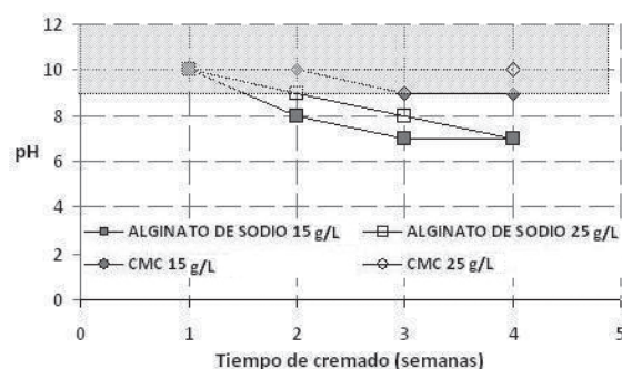
Figura 3. Relación entre el pH vs Tiempo de cremación para diferentes concentraciones de agente cremador.
