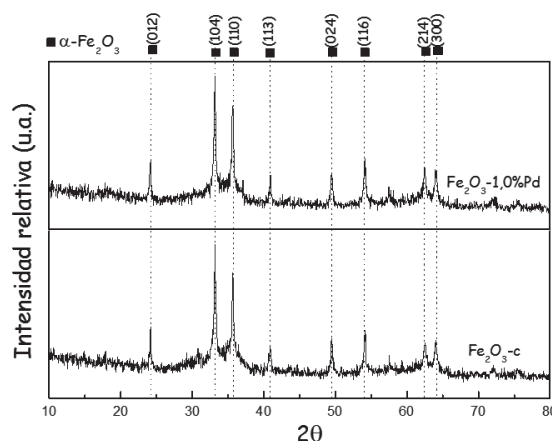
Figura 2. Efecto del dopante Pd en los difractogramas de las muestras basadas en nanopartículas de óxido de Fe. Muestra Fe 2 O 3 -1,0%p de Pd calcinada (arriba). Muestra Fe 2 O 3 -c (abajo).
