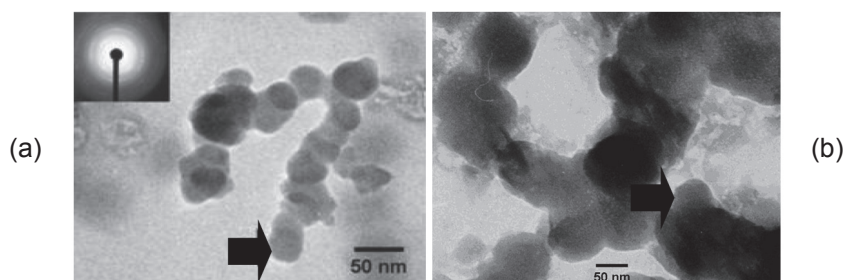
Figura 3. a: Microfotografía TEM de las nanopartículas de \text{Fe}_2\text{O}_3 -c sin dopar calcinadas a 400^\circ\text{C} . b: Microfotografía TEM de la muestra de \text{Fe}_2\text{O}_3 0,5%p de Pd dopada con cloruro de paladio.
