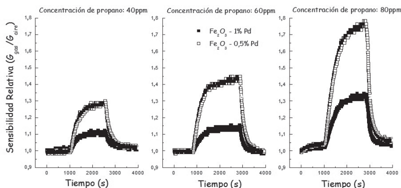
Figura 5. Comparación de la sensibilidad de los sensores basados en óxido de Fe dopados con 0,5 y 1,0%p de Pd a las concentraciones de 40, 60 y 80ppm de propano a la temperatura de 360^\circ\text{C} .
