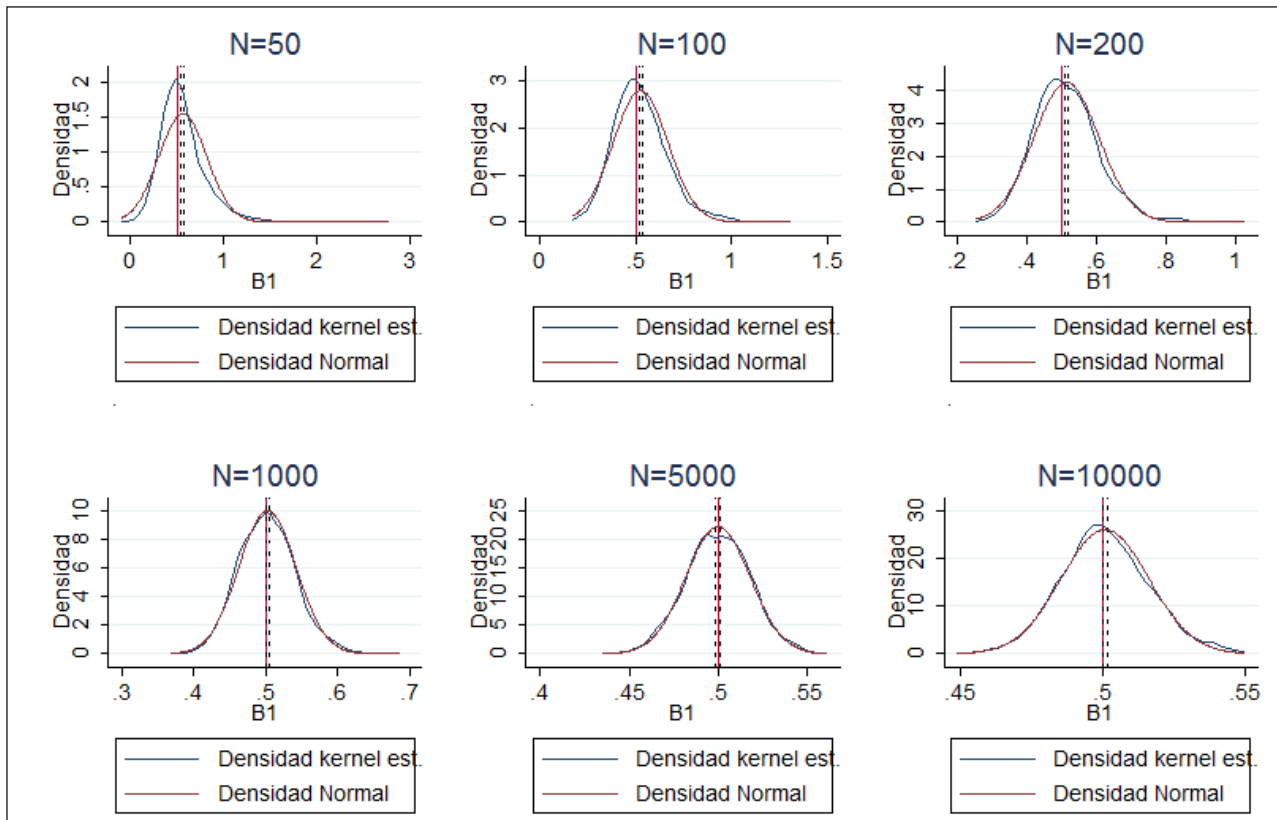
Figura 3. Modelo condicional estimado por Logit (proceso generador de datos normal)
