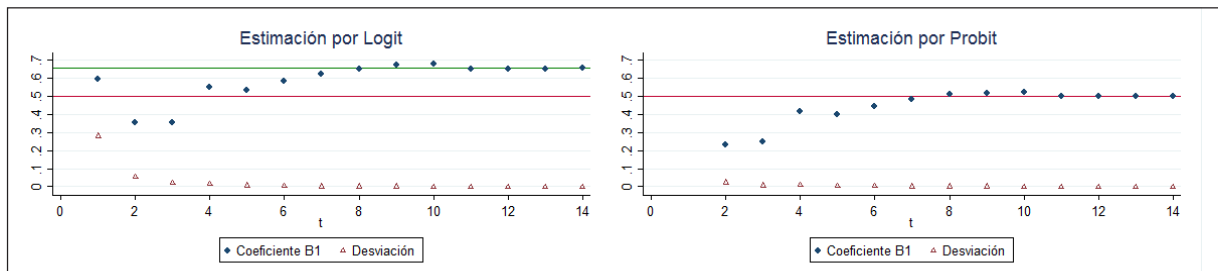
Figura 12. Consistencia modelo condicional (proceso generador de datos normal)
