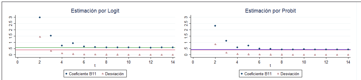
Figura 17. Consistencia modelo multinomial (proceso generador de datos t-student)
