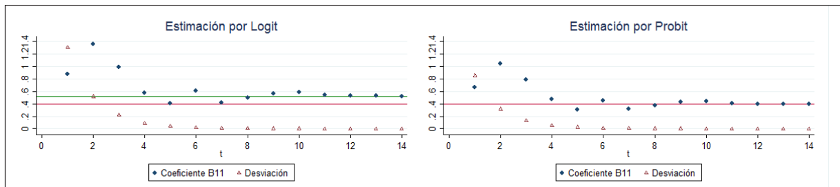
Figura 11. Consistencia modelo multinomial (proceso generador de datos normal)
