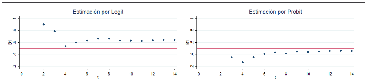
Figura 18. Consistencia del modelo condicional (proceso generador de datos t-student)
