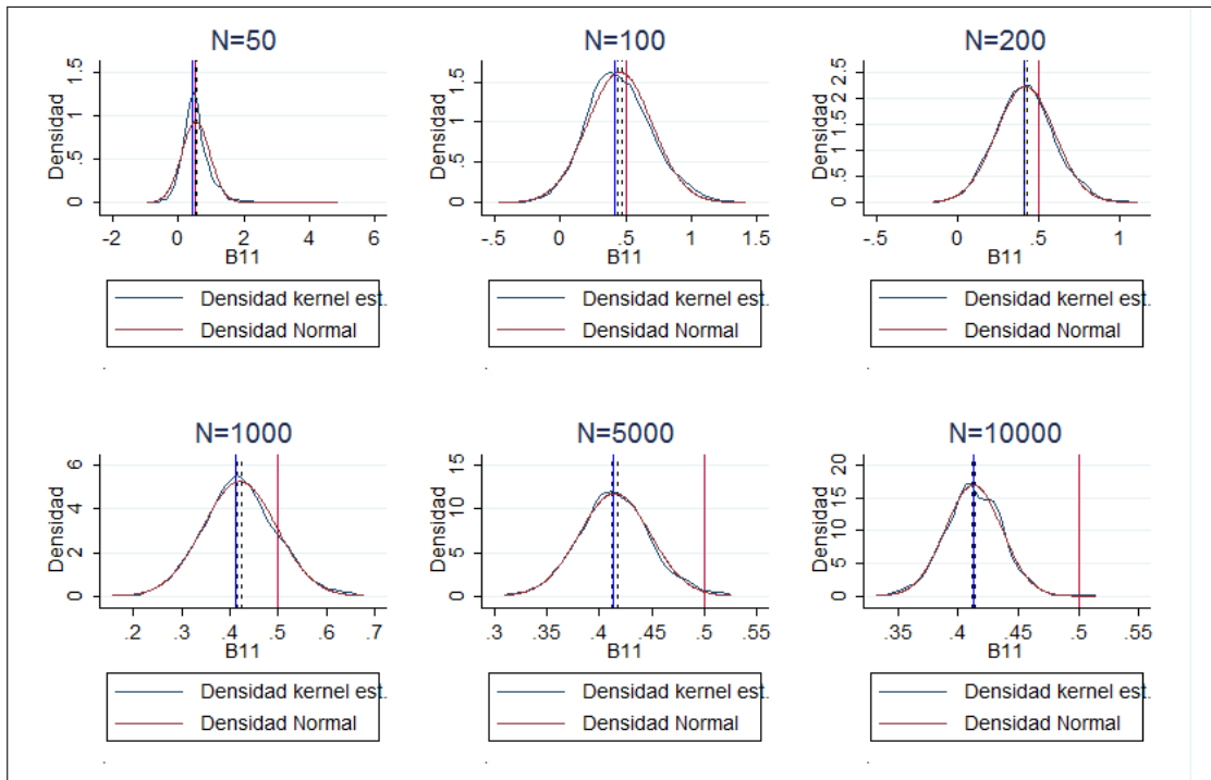
Figura 14. Modelo multinomial estimado por Probit (proceso generador de datos t-student)
