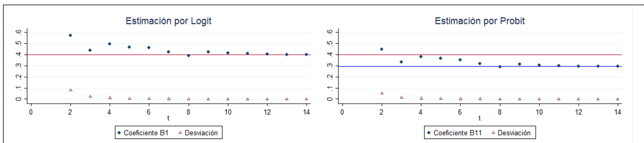
Figura 5. Aproximación a la propiedad de consistencia modelo multinomial (proceso generador de datos normal)
