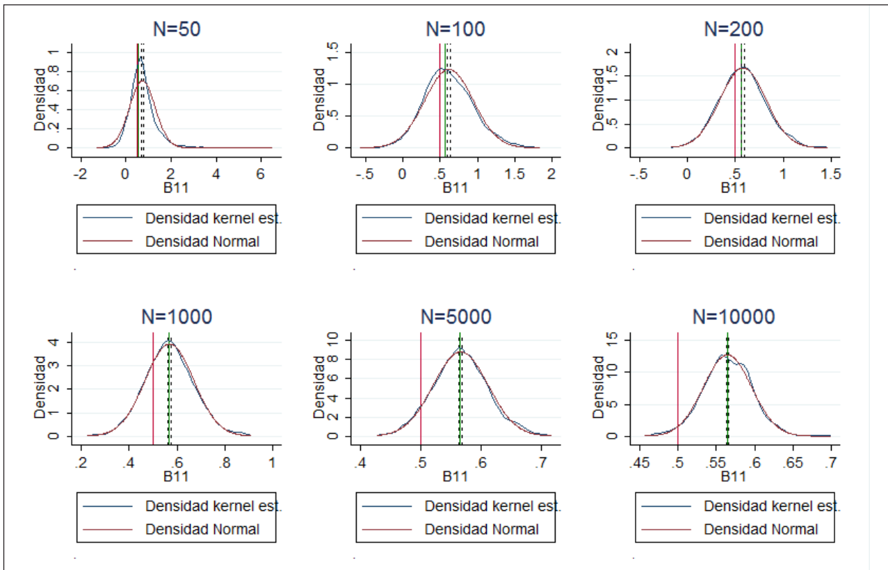
Figura 13. Modelo multinomial estimado por Logit (proceso generador de datos t-student)
