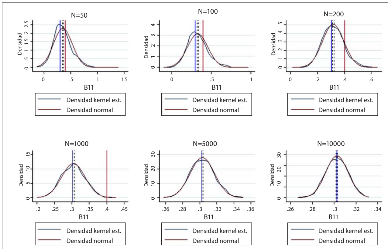
Figura 2. Modelo multinomial estimado por Probit (proceso generador de datos normal)
