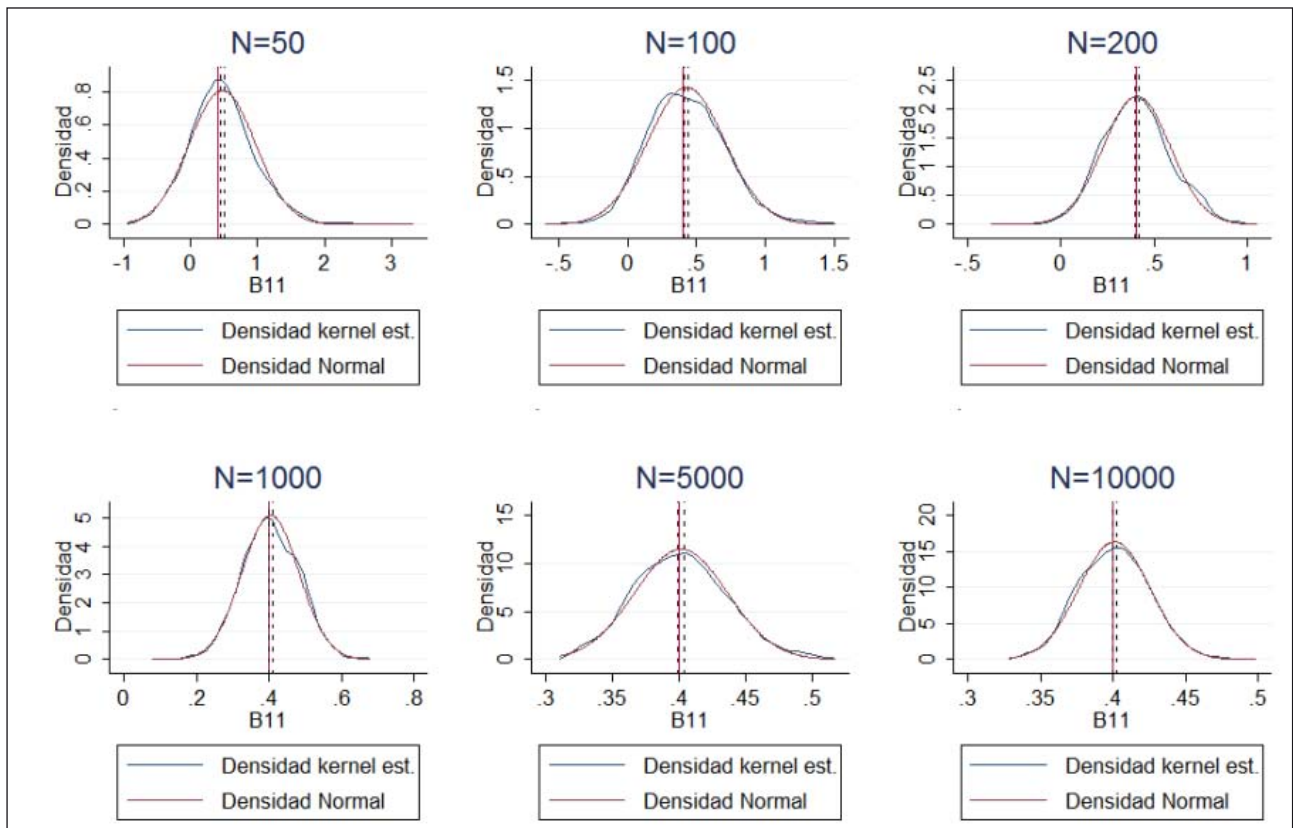
Figura 8. Modelo multinomial estimado por Probit (proceso generador de datos normal)
