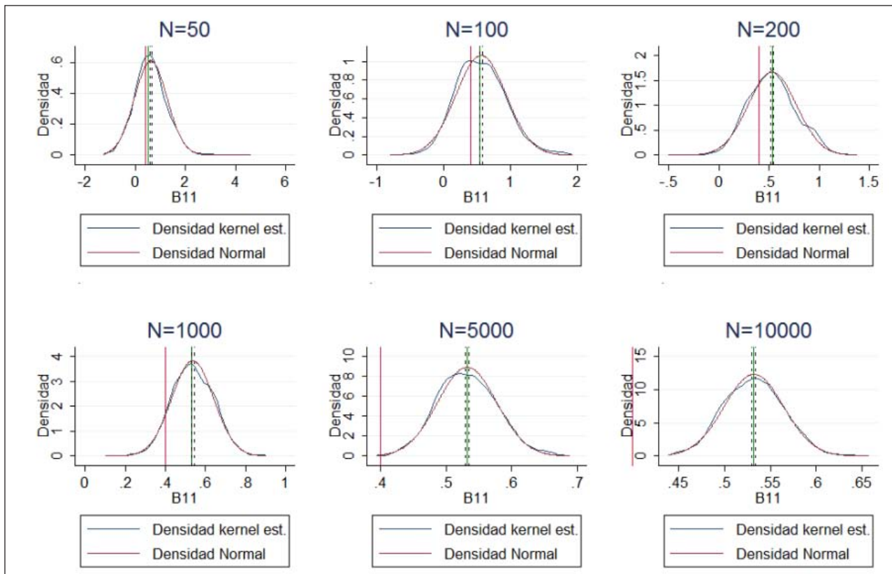
Figura 7. Modelo multinomial estimado por Logit (proceso generador de datos normal)
