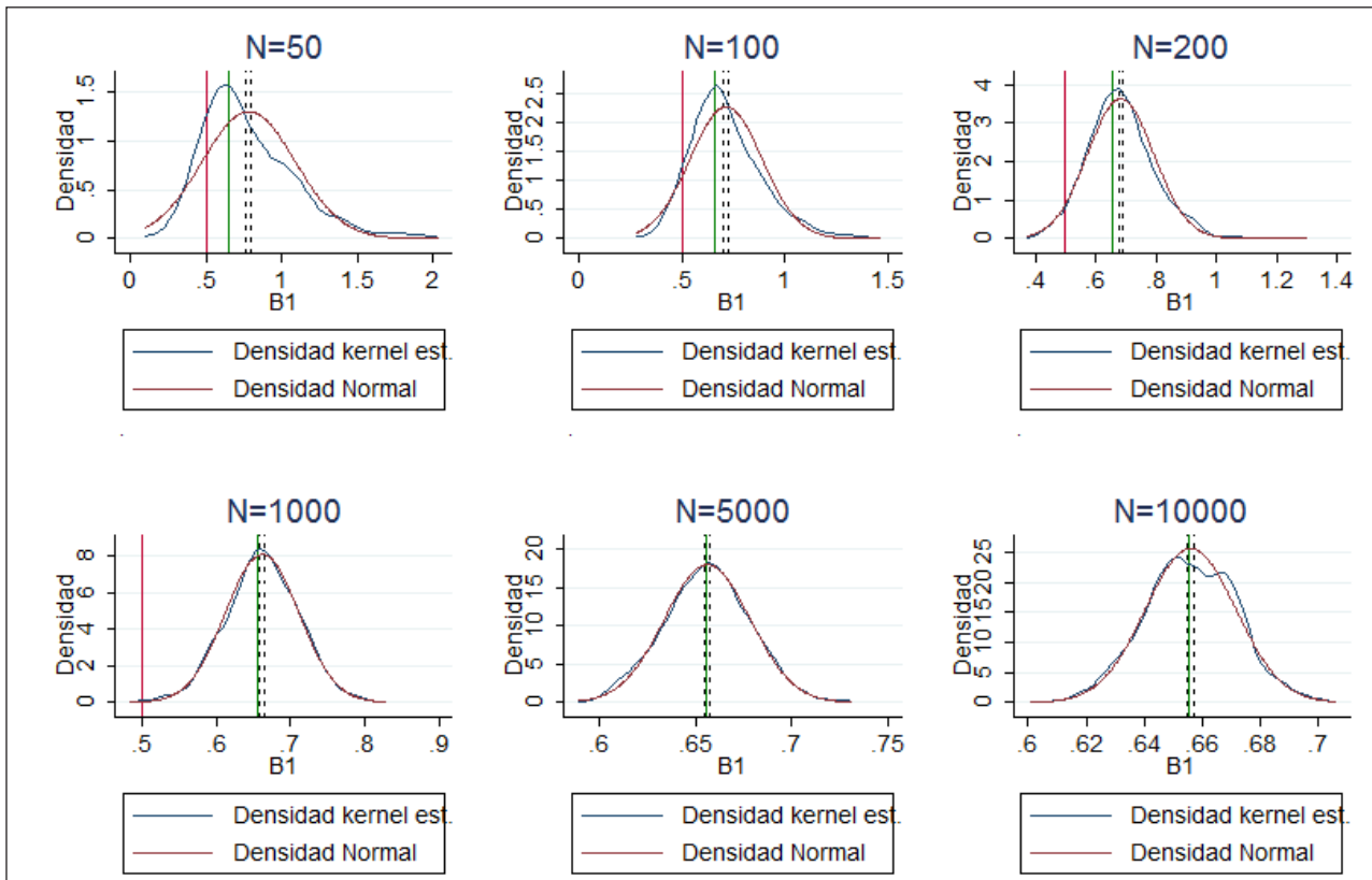
Figura 9. Modelo condicional estimado por Logit (proceso generador de datos normal)
