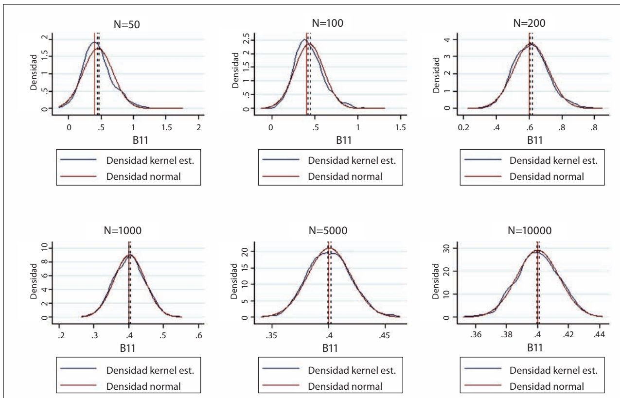
Figura 1. Modelo multinomial estimado por Logit (proceso generador de datos normal)
