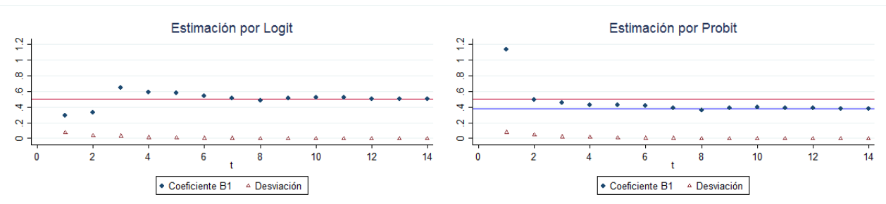
Figura 6. Aproximación a la propiedad de consistencia modelo Condicional (proceso generador de datos normal) Fuente: elaboración propia.
