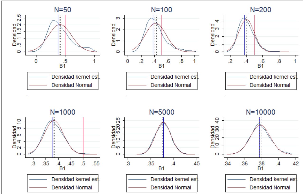
Figura 4. Modelo condicional estimado por Probit (proceso generador de datos logístico)
