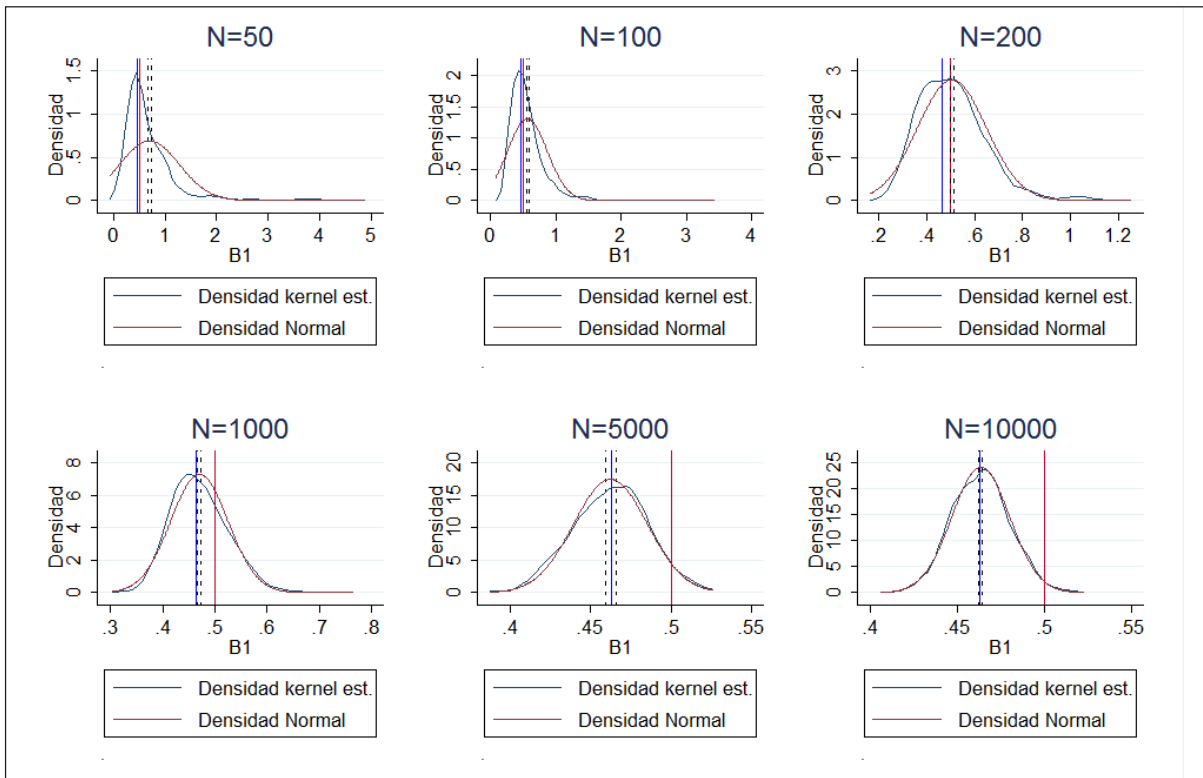
Figura 16. Modelo condicional estimado por Probit (proceso generador de datos t-student)
