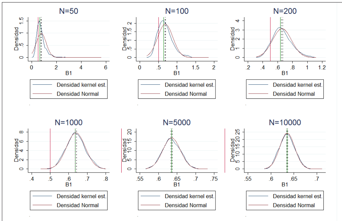
Figura 15. Modelo condicional estimado por Logit (proceso generador de datos t-student)
