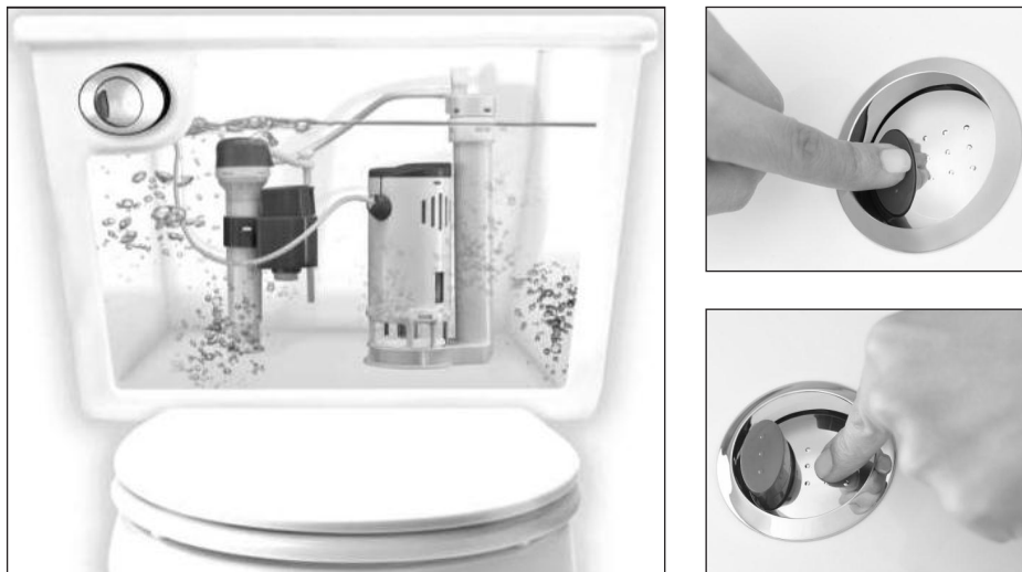
Figura 5. Sistema de doble descarga y regulador de volumen para inodoros.
