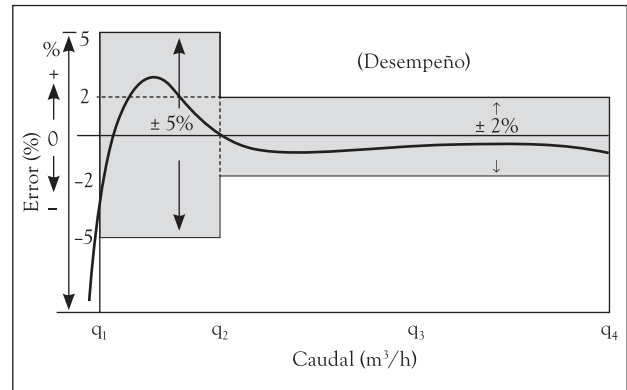
Figura 1. Curva característica medidor de agua potable.
