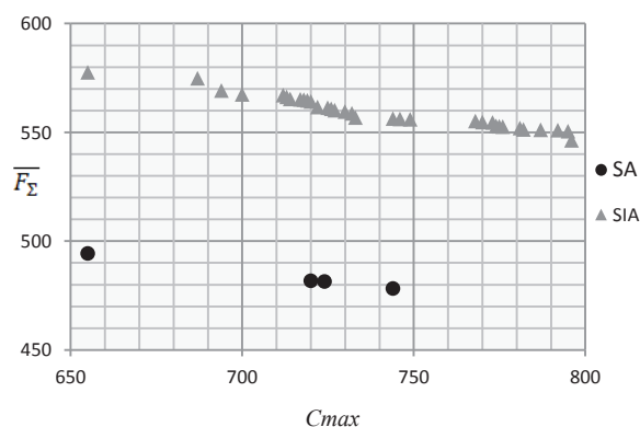
Figura 3. Frente de Pareto para el problema 10×5. (SA= algoritmo propuesto, SIA = Sistema inmune artificial [20])
