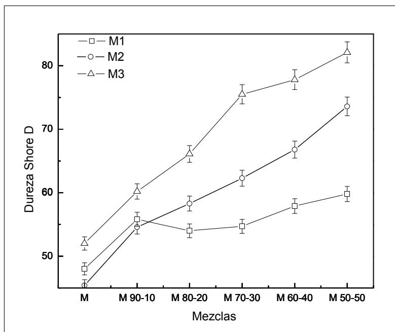
Figura 6. Variación de la dureza Shore D del Polietileno de baja densidad (M1), Polietileno de baja densidad lineal (M2) y Polipropileno post industrial de recorte de tela no tejidas (M3) mezclados con ceniza volante en porcentajes del 0 al 50 %.
