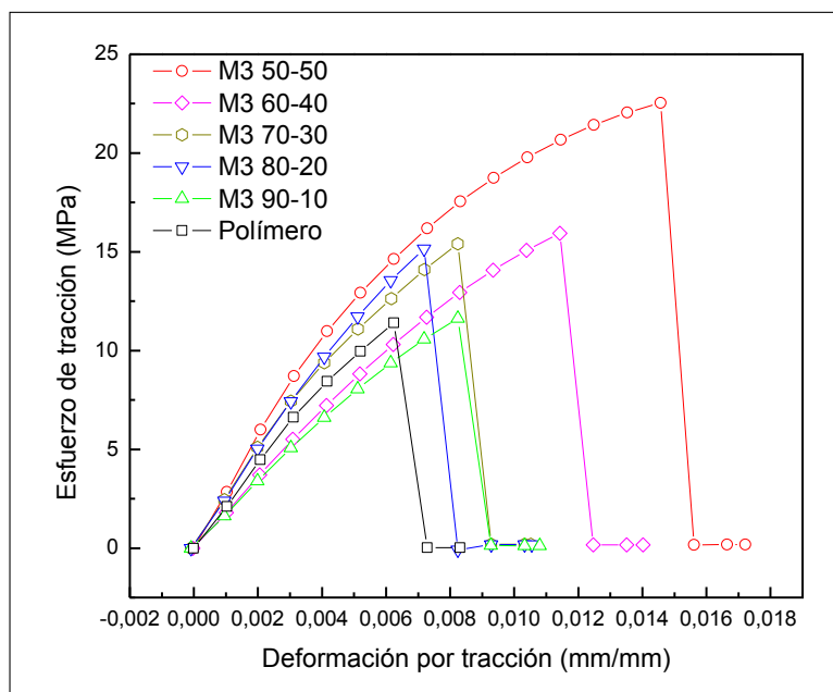
Figura 5. Polipropileno post industrial de recorte de tela no tejada mezclado con ceniza volante en porcentajes del 0 al 50 %.
