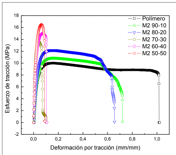
Figura 4. Polietileno de baja densidad lineal reciclado de los empaques de bolsas de leche, mezclado con ceniza volante en porcentajes del 0 al 50 %.
