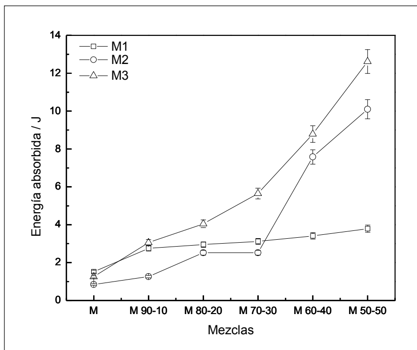
Figura 7. Variación de la energía absorbida del Polietileno de baja densidad (M1), Polietileno de baja densidad lineal (M2) y polipropileno post industrial de recorte de tela no tejidas (M3) mezclados con ceniza volante en porcentajes del 0 al 50 %.
