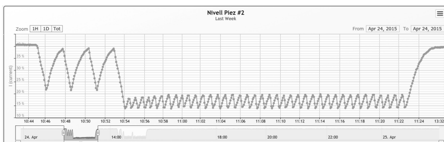
Figura 13. La plataforma permite la realización de gráficas de operación en tiempo real de cada uno de los elementos del sistema para facilitar la toma de decisiones.
