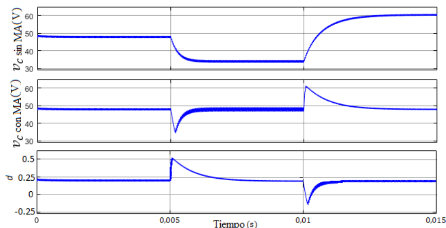
Figura 7. Tensión de salida sin mecanismo adaptativo (arriba) y con mecanismo adaptativo (abajo) frente a tres cambios de carga tipo paso
