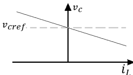
Figura 1. Corriente del SAE de acuerdo con la tensión del bus DC
