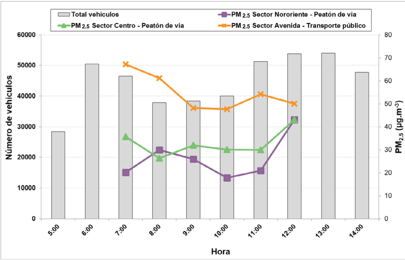
Figura 4. Relación entre las concentraciones promedio horarias halladas para PM_{2.5} y el comportamiento horario de tráfico vehicular en la ciudad de Manizales, los datos de distribución vehicular se tomaron del estudio de movilidad de la ciudad [9].
