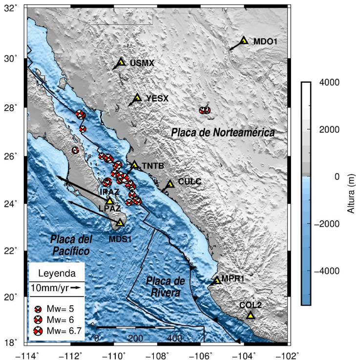
Figura 5. Campo de velocidad obtenido a través de la estimación de las velocidades residuales con respecto al marco de referencia ITRF14 de la placa de Norteamérica creada a partir de la tabla 2 con un intervalo de confianza de 95 %. Imagen a color con relieve sombreado extraído del Modelo Relieve Global de ETOPO1 [25].
