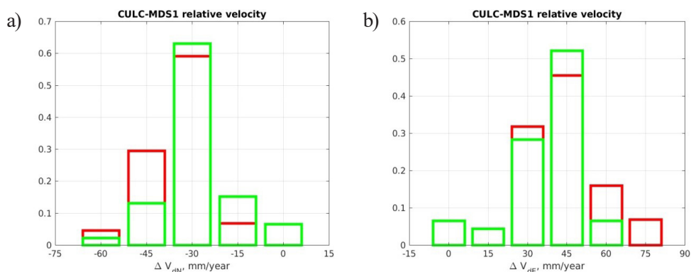
Figura 6. Distribución de velocidades de movimiento relativo entre las estaciones "CULC" y "MDS1" calculadas cada 55 días (verde) y 55 días antes del sismo (rojo): (a) componente norte, (b) componente este.
