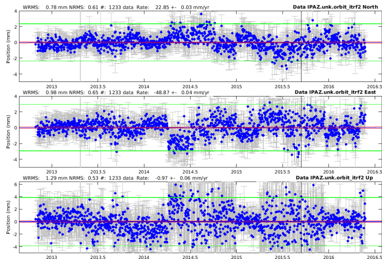
Figura 4. Series temporales de posiciones (n, e, u) de IPAZ ajustadas. Puntos azules: Posiciones diarias respecto a la posición de referencia en sus tres componentes neu. De arriba hacia abajo: norte, este y vertical. Líneas rojas: corresponden a las incertidumbres realistas ( \pm 1\sigma ) estimadas. Líneas verdes: error medio cuadrático ponderado de cada componente en mm ( \pm 3 la dispersión).
