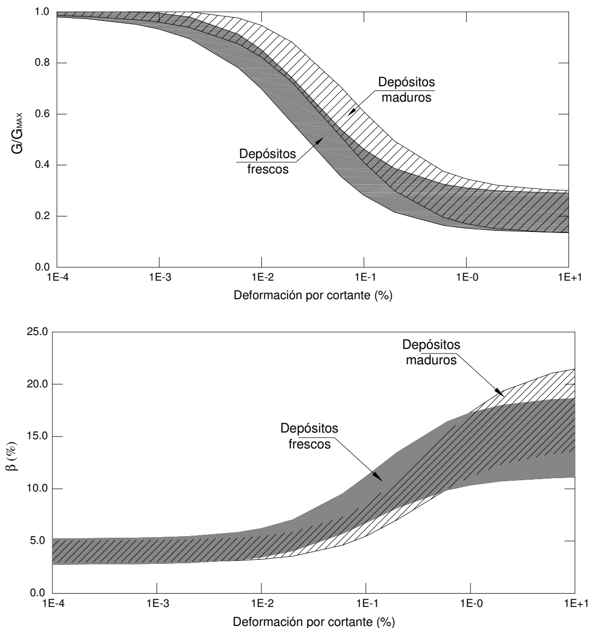
Figura 2. Bandas propuestas para la degradación del modulo de rigidez a cortante y amortiguamiento en los suelos trasportados de Gabro.
