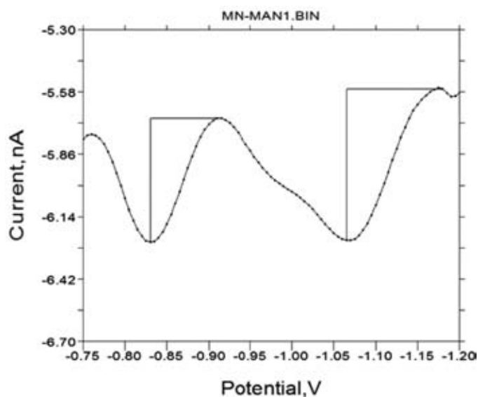
Figura 1. Voltametría lineal para reducción de Zinc ( -860\text{ mV} ) y Manganeso ( -1100\text{ mV} ).
