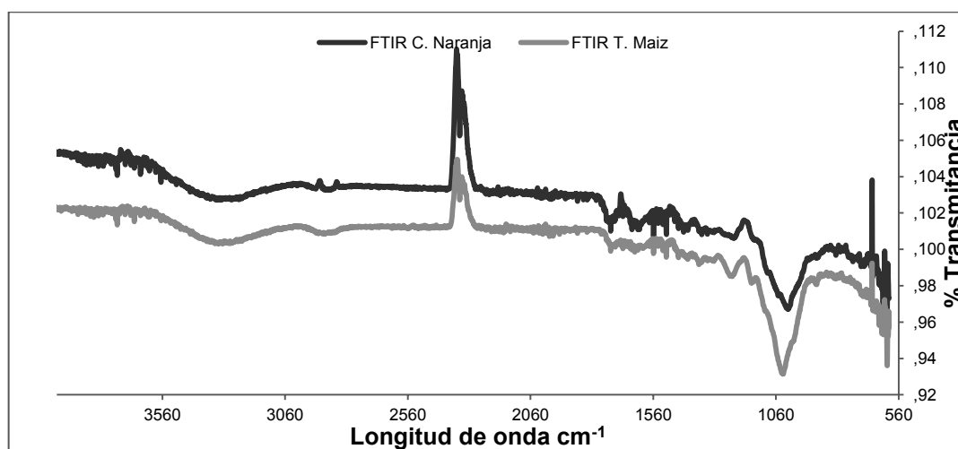
Figura 1. Espectrofotometría de infrarrojo de la cáscara de naranja y zurro de maíz, antes del proceso de adsorción de Pb (II).
