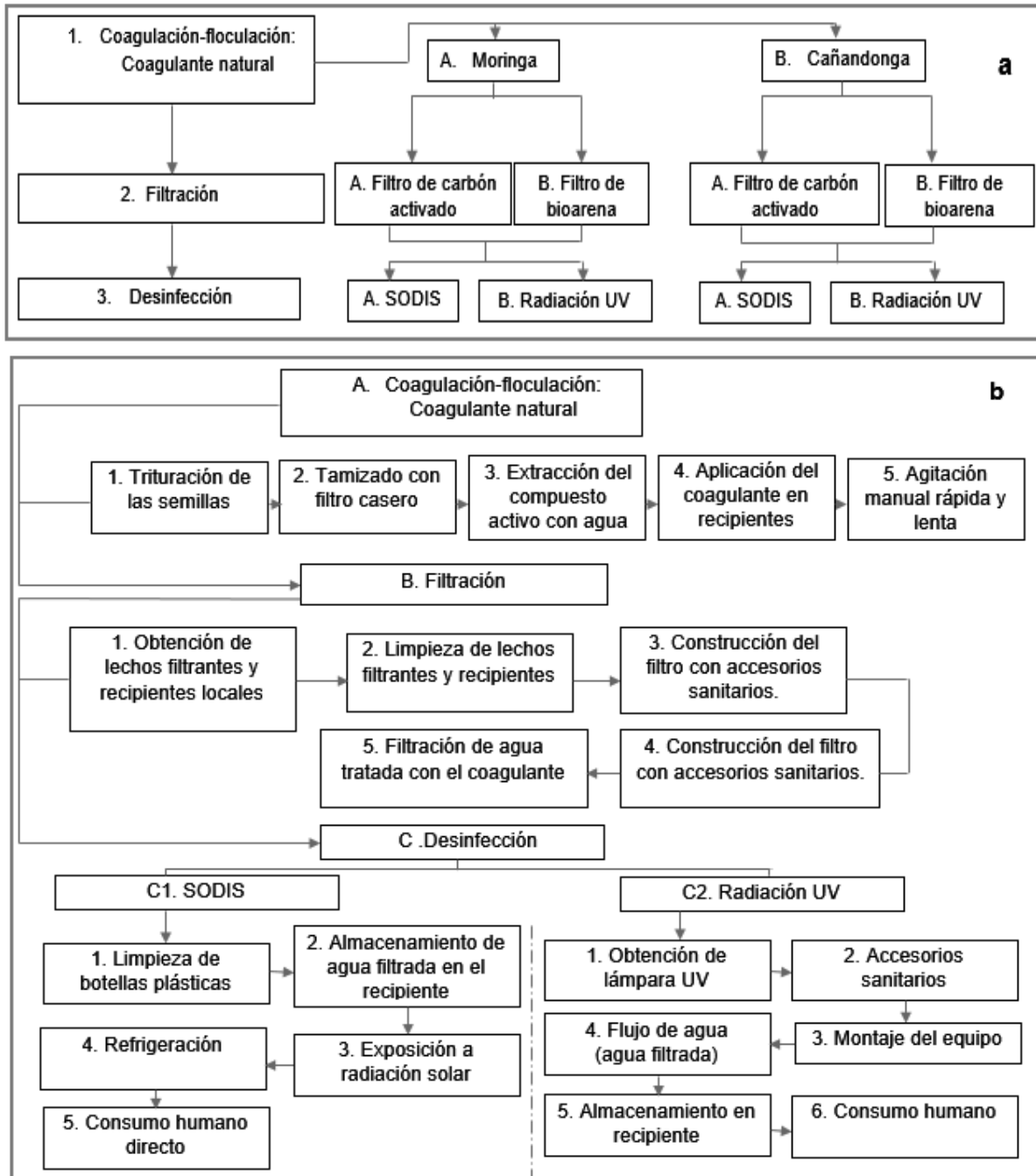
Figura 1. (a) Diagrama general de los procesos propuestos para la potabilización no convencional (artesanal) y (b) Esquema general del procedimiento de purificación de agua en los pueblos palafíticos: Nueva Venecia y Buena Vista.
