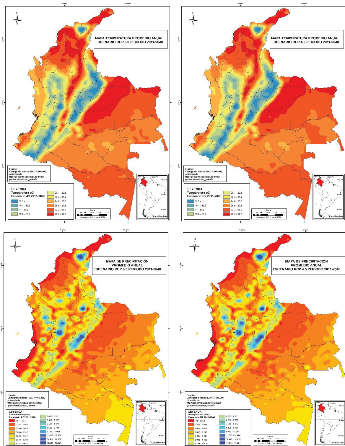
Figura 3. Temperatura media anual del aire (arriba) y precipitación anual (abajo), bajo los escenarios RCP 4,5 y 6,0, periodo 2011-2040.
