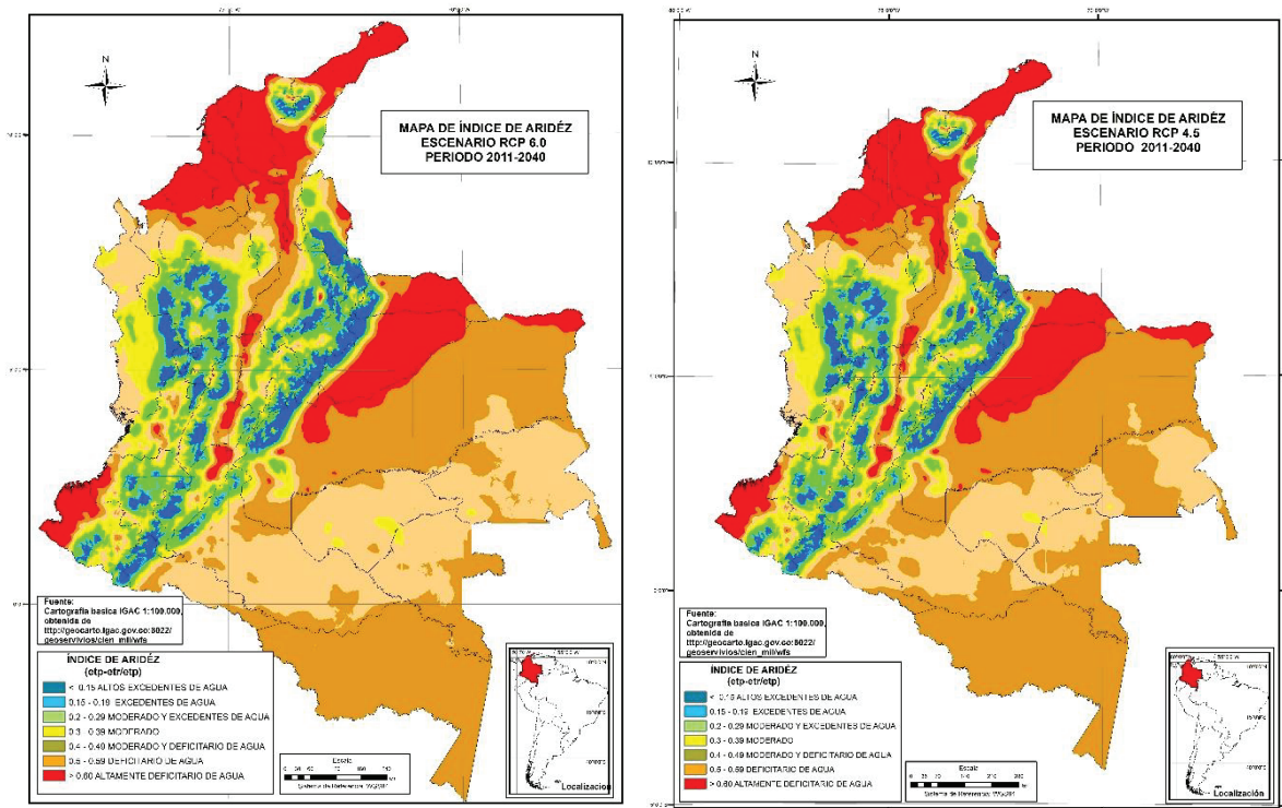
Figura 5. Distribución potencial del índice de aridez bajo los escenarios 6,0 y 4,5, periodo 2011-2040.
