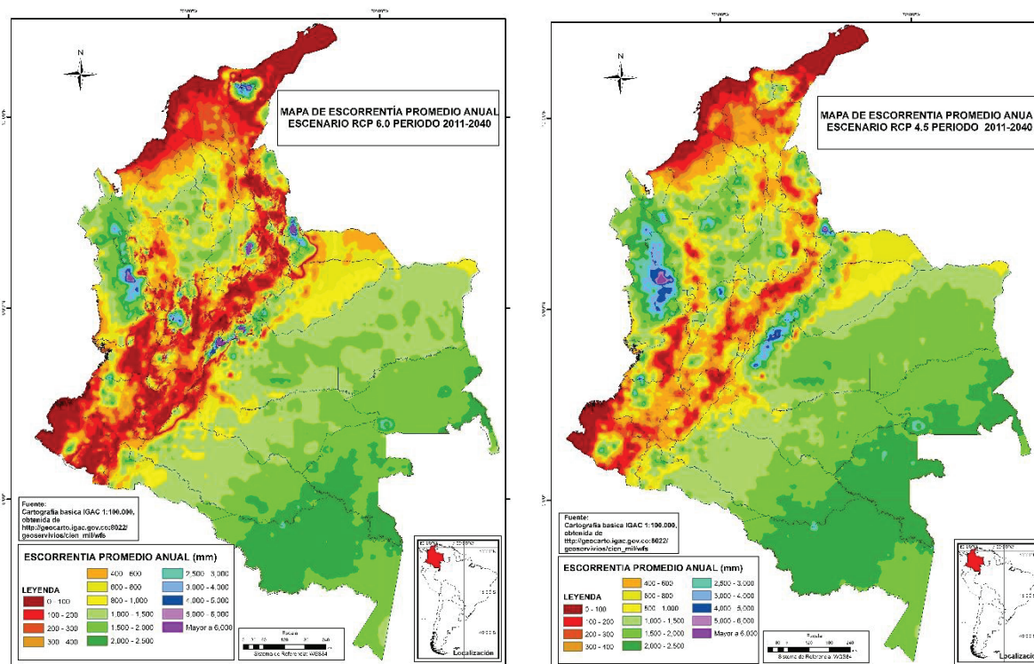
Figura 4. Distribución potencial de la escorrentía bajo los escenarios 6,0 y 4,5, periodo 2011-2040.
