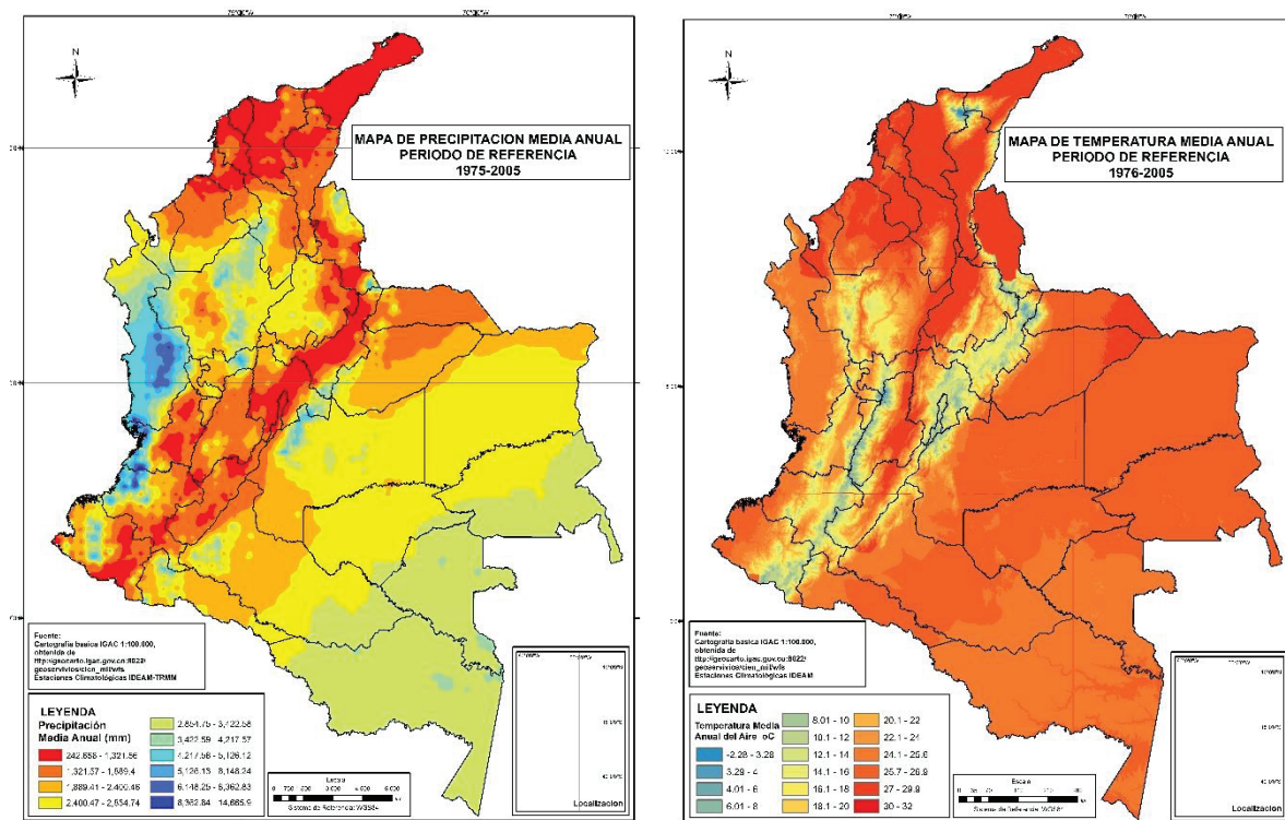
Figura 1. Mapa de precipitación media anual y temperatura media anual del aire periodo de referencia 1976-2005.
