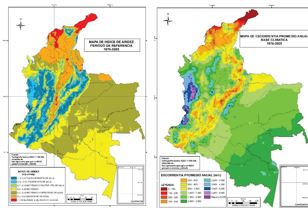
Figura 2. Mapa de escorrentía promedio anual (izquierda) e Índice de Aridez (derecha), periodo de referencia 1976-2005.
