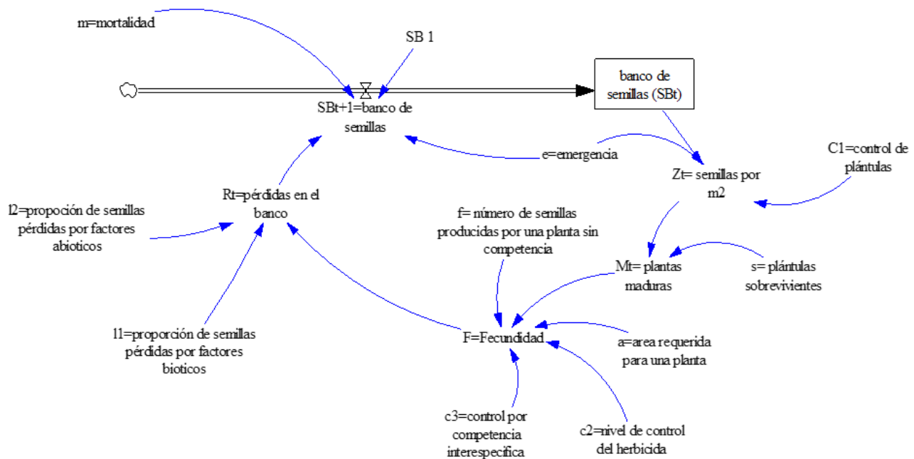
Figura 1. Diagrama de Forrester, que incluye las variables comprendidas en la construcción del modelo m 2 .
