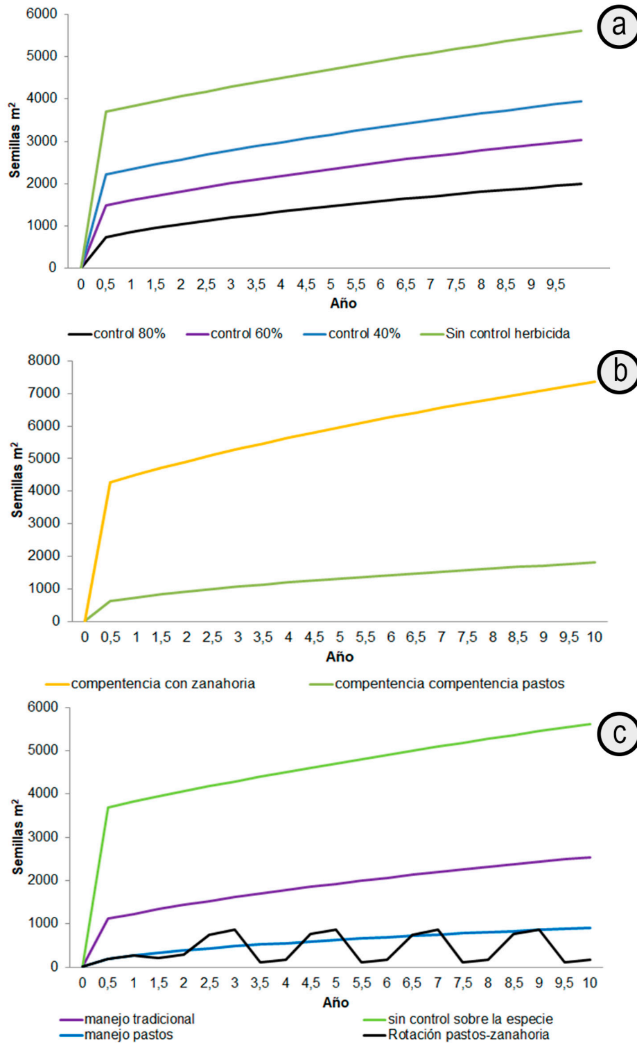
Figura 2. Modelación según cada uno de los escenarios: a. proyección del Banco de semillas de S. vulgaris con la aplicación de herbicidas, en cuatro escenarios-control; b. proyección del Banco de semillas de S. vulgaris en competencia interespecífica, con siembra de pasturas y con zanahoria; c. proyección del Banco de semillas de S. vulgaris cuando se implementa un modelo de manejo integrado de la población de S. vulgaris .
