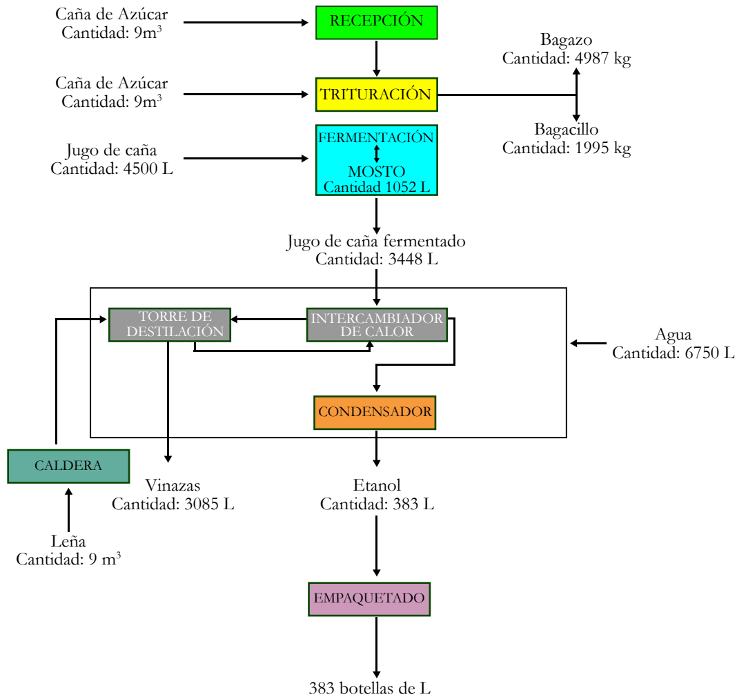
Figura 1. Diagrama de flujo del proceso productivo de la destilería “Rivera Revilla Fray Ángel”, para 383 botellas de 1 L.
