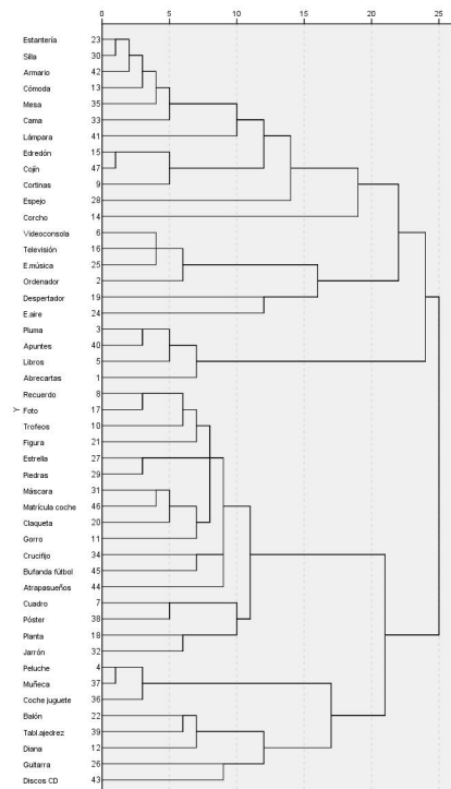
Figura 1 Representación gráfica de las agrupaciones de los objetos obtenidas por el análisis de cluster
