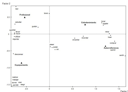
Figura 2 Análisis de correspondencia simple entre verbos y categorías
