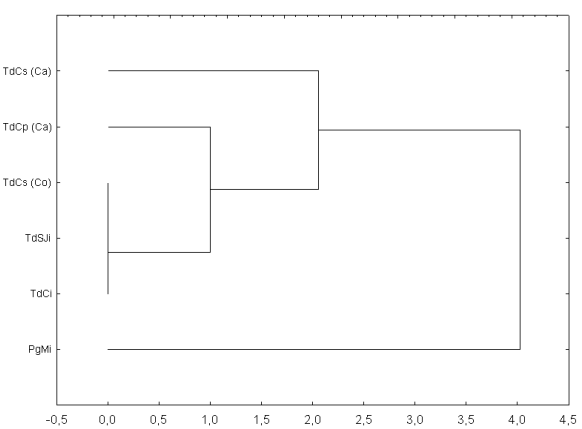
Figura 2. Fenograma construido por el método UPGMA ( Unweighted Pair Group Method Analysis ) usando distancias euclidianas, de perfiles electroforéticos de las proteínas salivares de T. dimidiata : TdCi (Capitanejo, intradomicilio, colonia), TdSji (San Joaquín, intradomicilio, colonia), TdCs (Co) (Capitanejo, silvestre, colonia), TdCp (Ca) (Capitanejo, peridomicilio, campo), TdCs (Ca) (Capitanejo, silvestre, campo). Y P. geniculatus : PgMi (Molagavita, intradomicilio, colonia).
