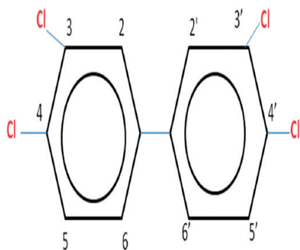
Figura 1. Derivado del bifenilo. Estructura del 3,3', 4,4' - tetrachlorobifenil (PBC-77)
