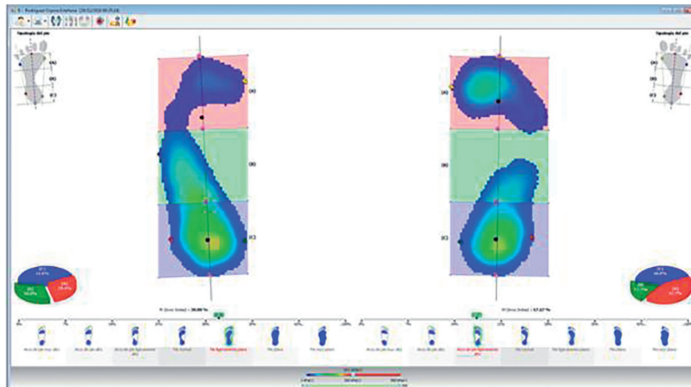
Figura 3. Tipología plantar.
