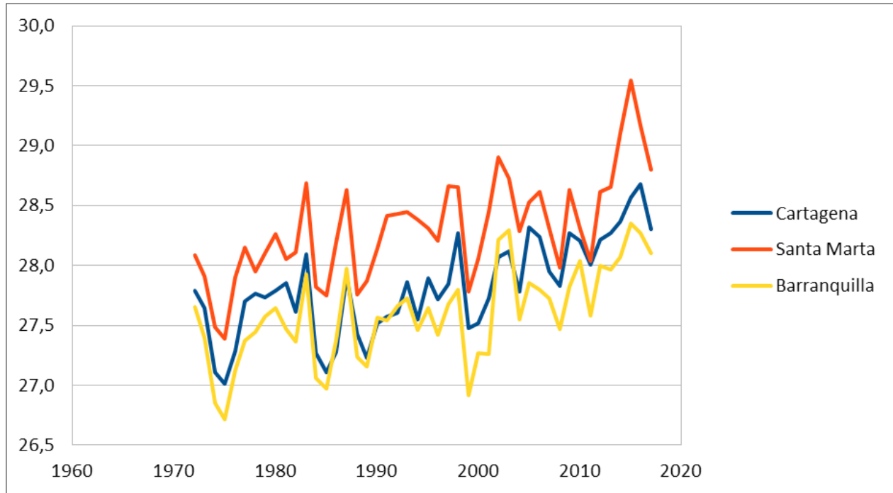
Figura 1. Evolución de la temperatura media anual en el Caribe colombiano entre 1972 y 2017
