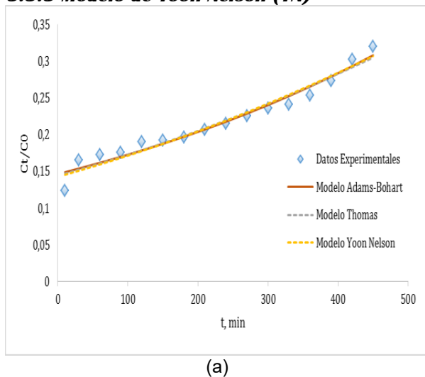
Fig. 3 (a). Ajuste de los modelos cinéticos de adsorción de Hg(II) de la columna empacada con de 4 cm (a) y 7.5 cm(b)
