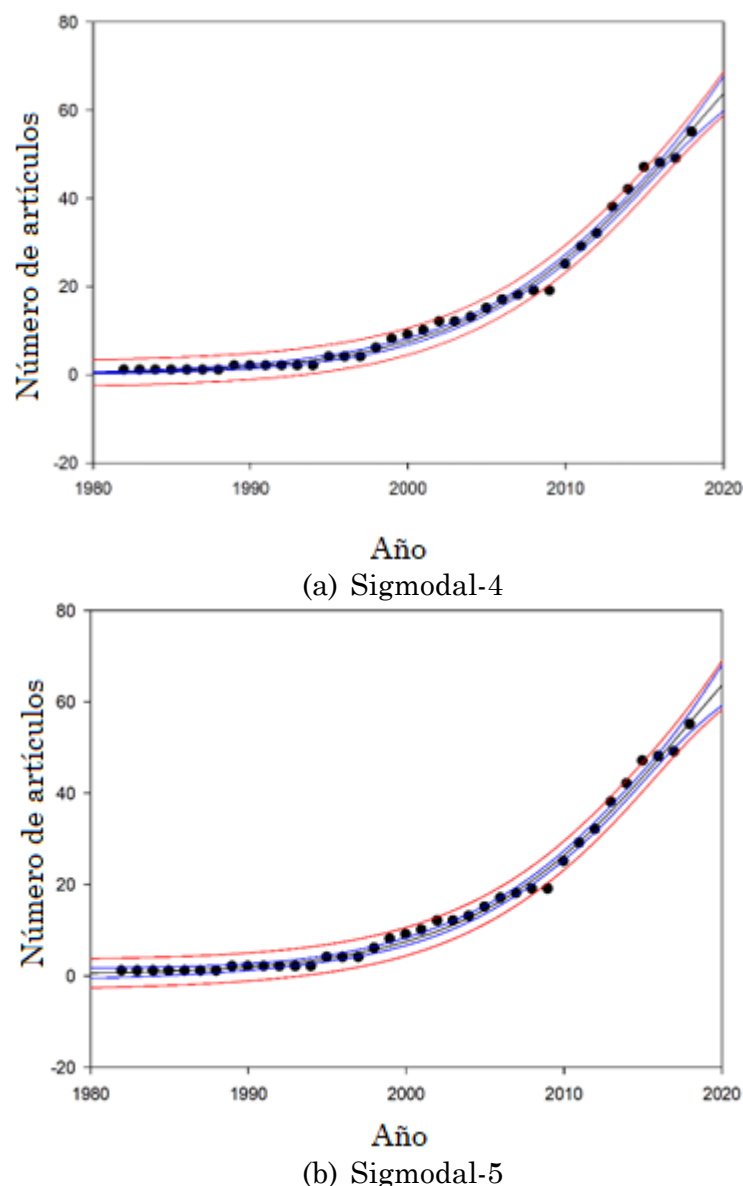
Fig. 4. Curva en S de mejor ajuste estadístico para artículos de la ecuación ATK ( Amaranthus AND climate). Fuente: autores.
