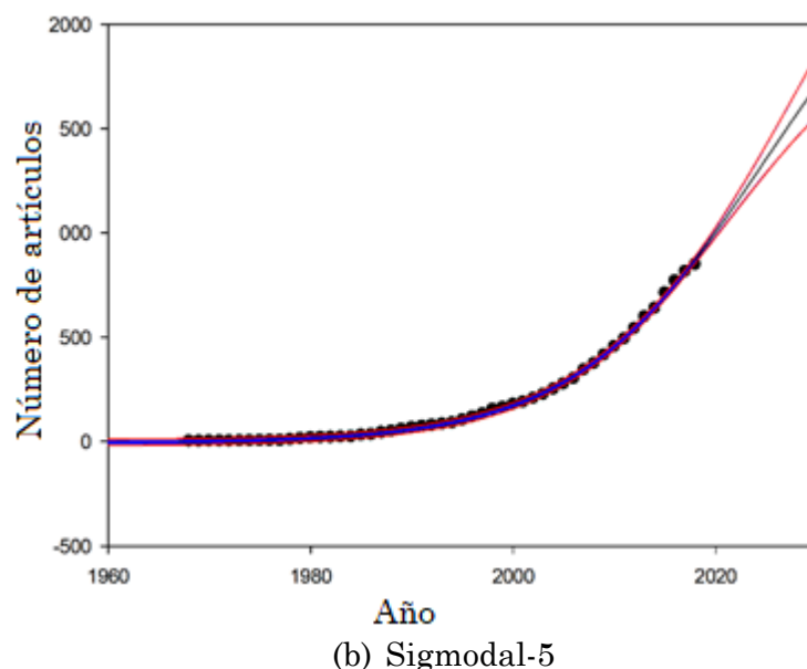
Fig. 3. Curva en S de mejor ajuste estadístico para artículos de la ecuación ATK ( Amaranthus AND food). Fuente: autores.
