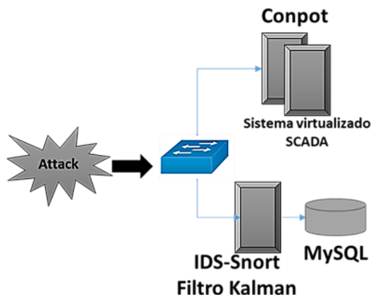
Fig. 3. Arquitectura de implementación Fuente: elaboración propia.
