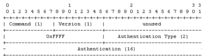
Figura 8. Esquema de autenticación.
