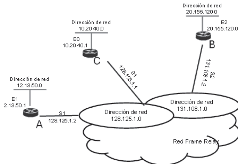
Figura 12. Escenario de configuración de RIP.
