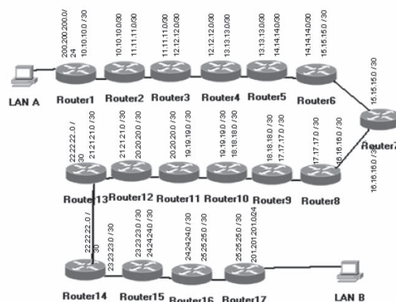
Figura 16. Escenario y configuración de enrutadores.
