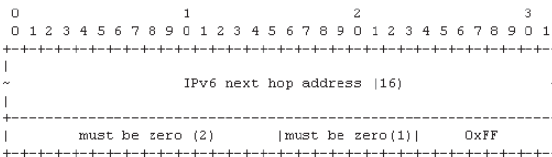
Figura 11. Formato del próximo salto de ruta.
