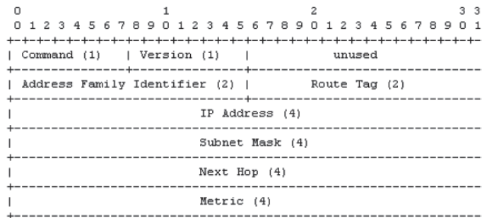
Figura 7. Nuevo formato del mensaje RIP.
