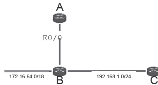
Figura 13. Esquema de una red.
