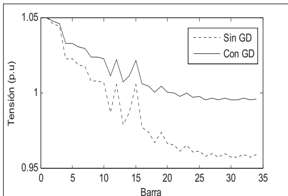
Fig. 6. Perfil de tensiones con y sin GD.
