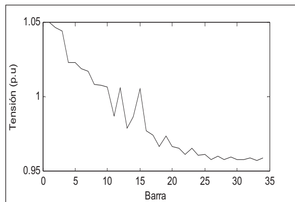
Fig. 4. Perfil de tensiones del sistema sin GD.
