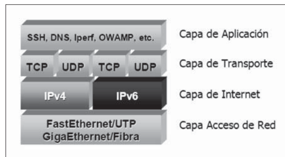
Figura 1. Modelo TCP/IP Double Stack
