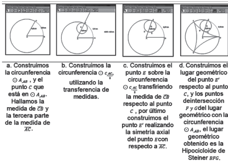
Figura 8. Hipocicloide de Steiner BFG
