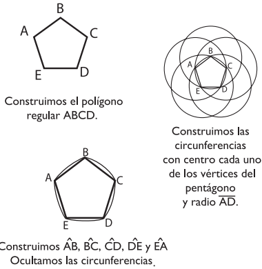
Figura 5. Pentágono de ancho constante
