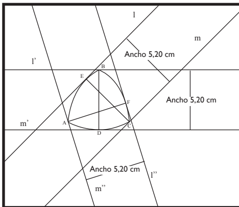
Figura 1. Diagrama de ancho constante. Triángulo de Relaux
