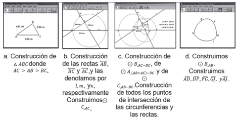
Figura 14. Figura de ancho constante a partir de un triángulo escaleno
