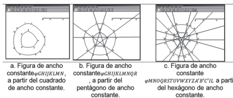
Figura 13. Figuras de ancho constante a partir de otra figura de ancho constante
