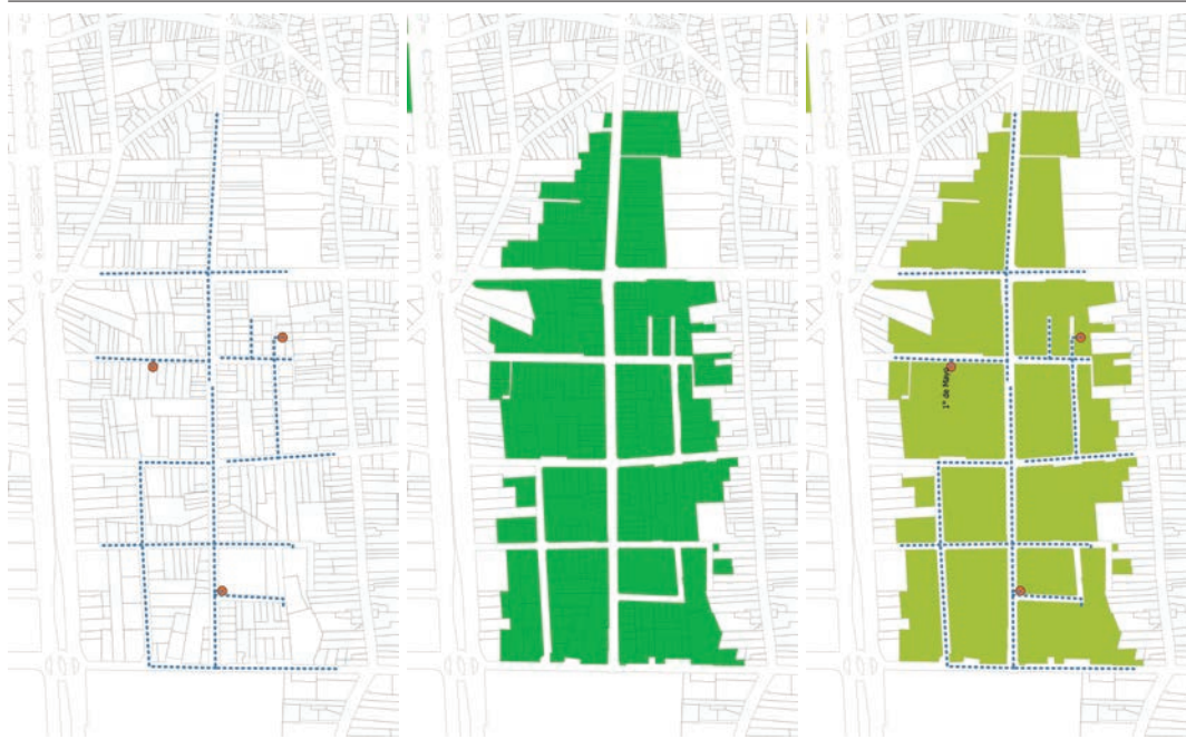
Figura 4. Relación entre estructura de red OLPE y forma del barrio
